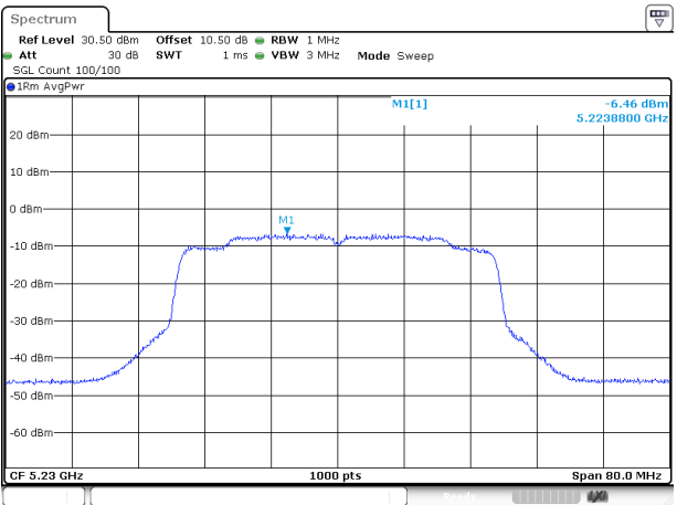
802.11ac40_5230MHz_ANT 2
