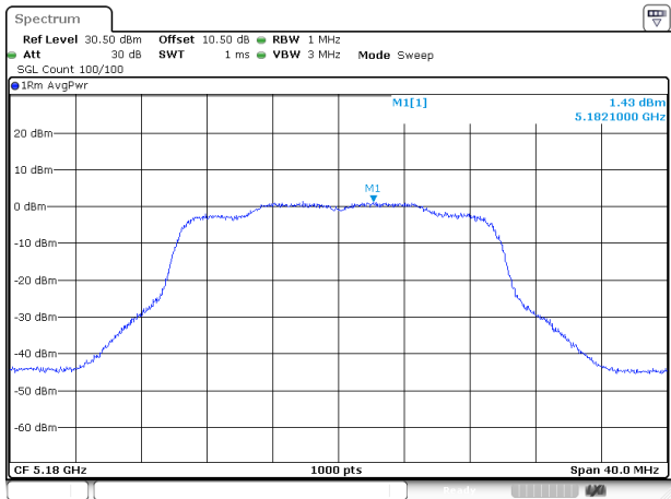
802.11ac20_5180MHz_ANT 1
