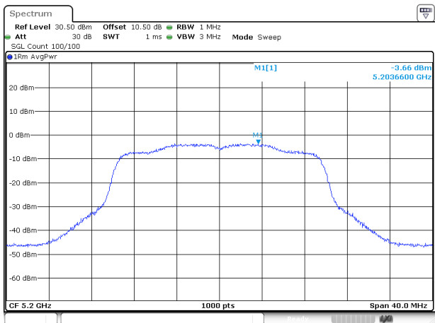
802.11ac20_5200MHz_ANT 2
