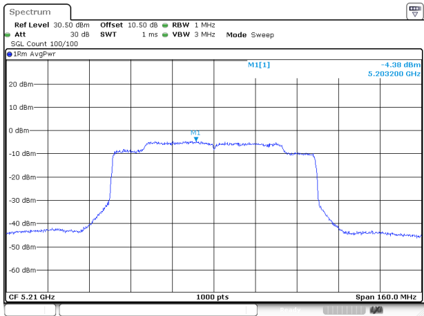
802.11ac80_5210MHz_ANT 1
