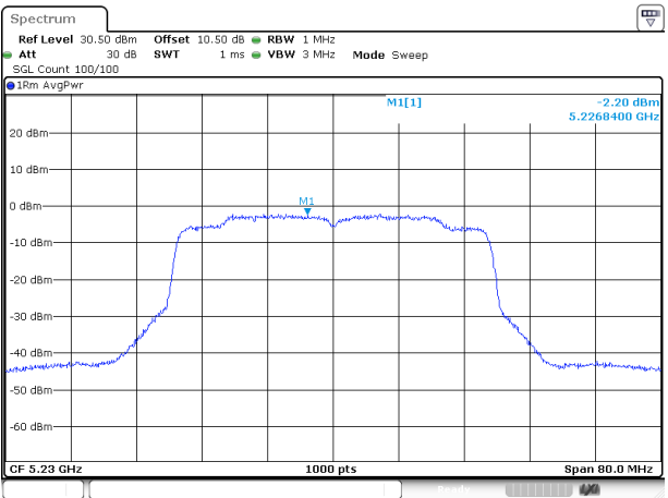
802.11ac40_5230MHz_ANT 1
