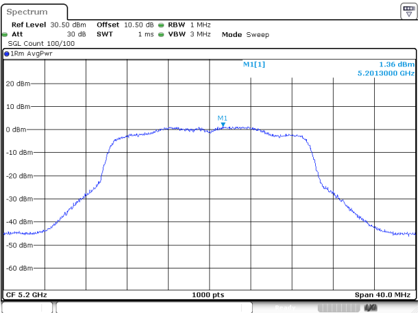
802.11ac20_5200MHz_ANT 1
