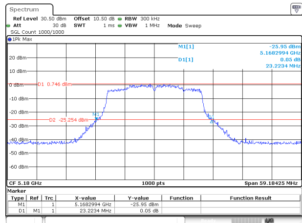
802.11ac20_5180MHz_ANT 2
