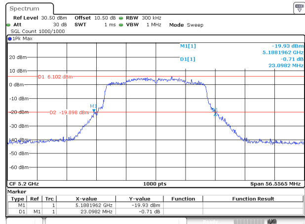
802.11ac20_5200MHz_ANT 1
