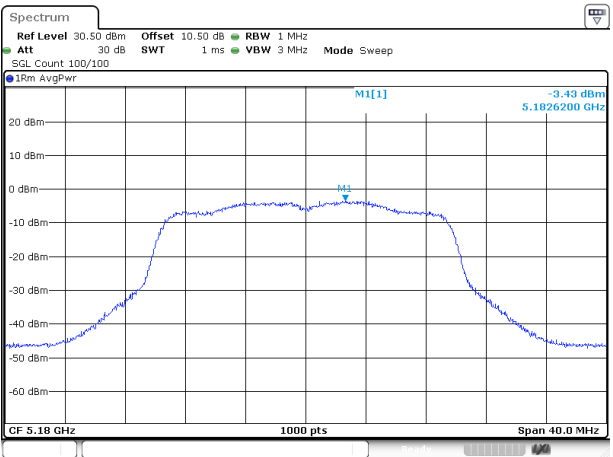
802.11ac20_5180MHz_ANT 2
