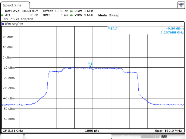
802.11ac80_5210MHz_ANT 2
