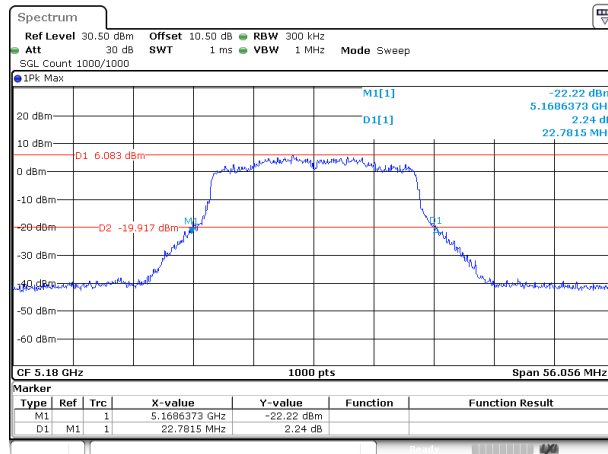
802.11ac20_5180MHz_ANT 1
