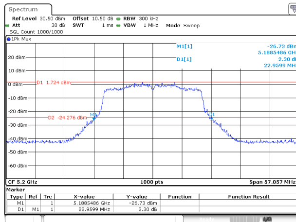
802.11ac20_5200MHz_ANT 2
