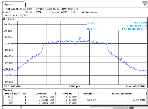
802.11n20_2462MHz_ANT 2
