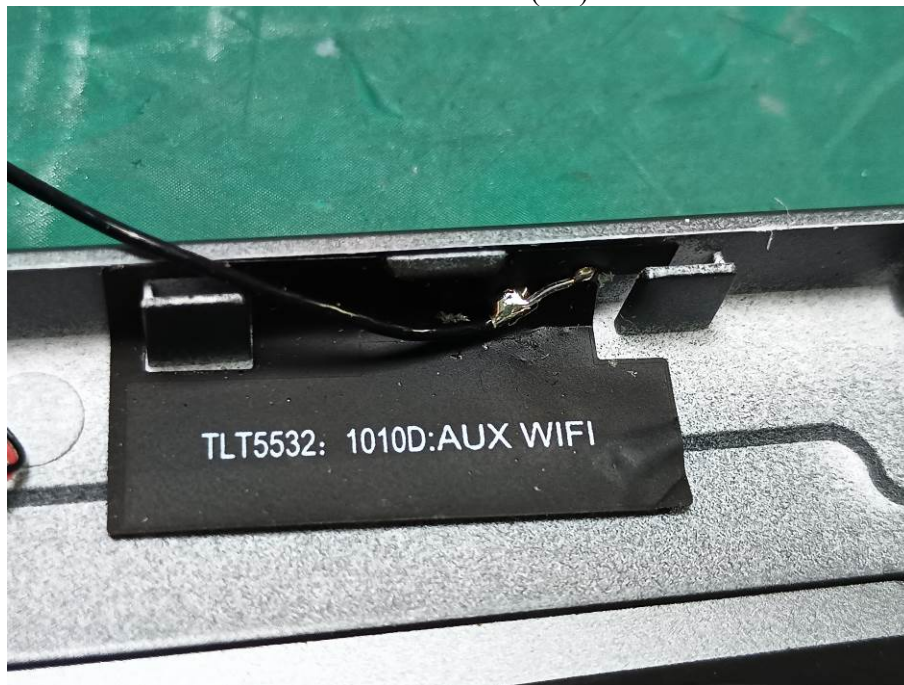
BT/ Wi-Fi ANT (TX)
