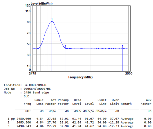
BLE_2M_TX_CH_39_Horizontal-Avg
