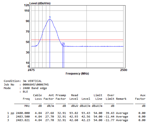
BLE_2M_TX_CH_39_Vertical-Avg
