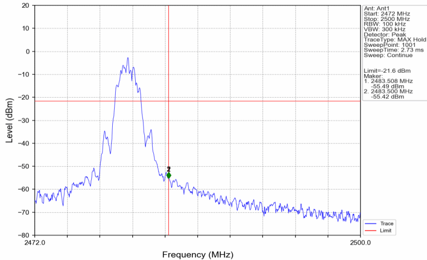
2M_HCH_2480MHz_Ant1_NTNV
