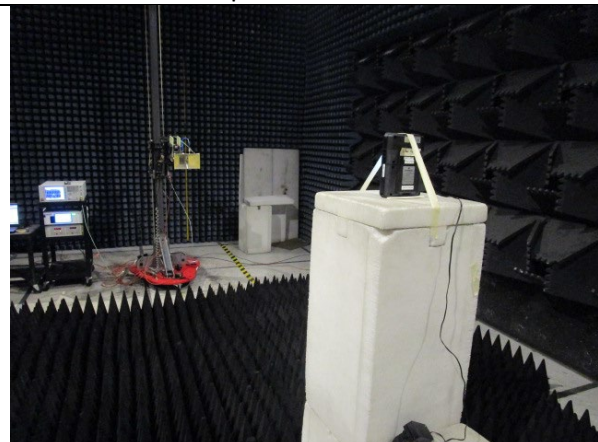
4-18GHz setup
