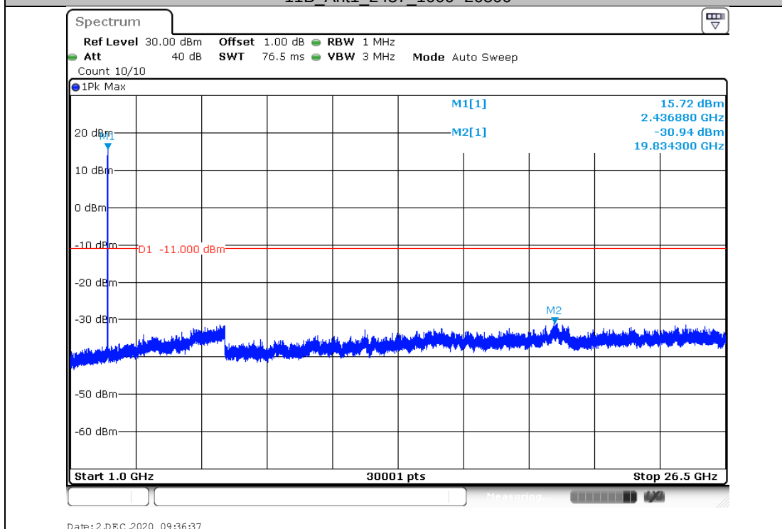
11B_Ant1_2437_1000~26500
