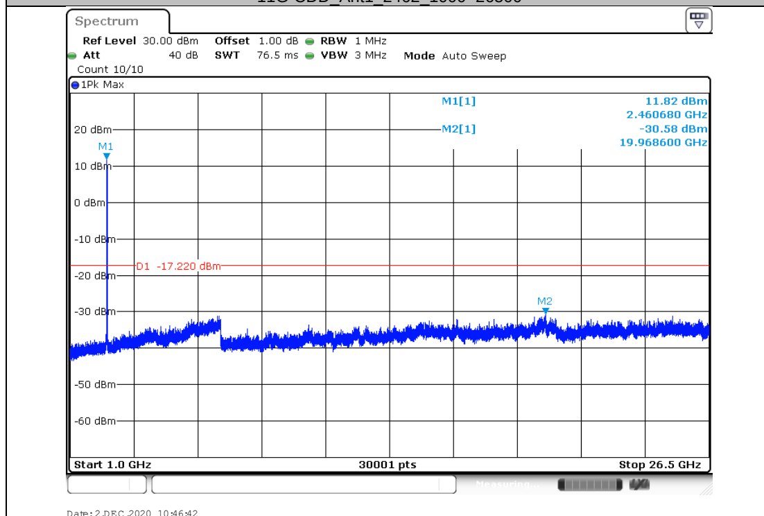
11G-CDD_Ant1_2462_1000~26500
