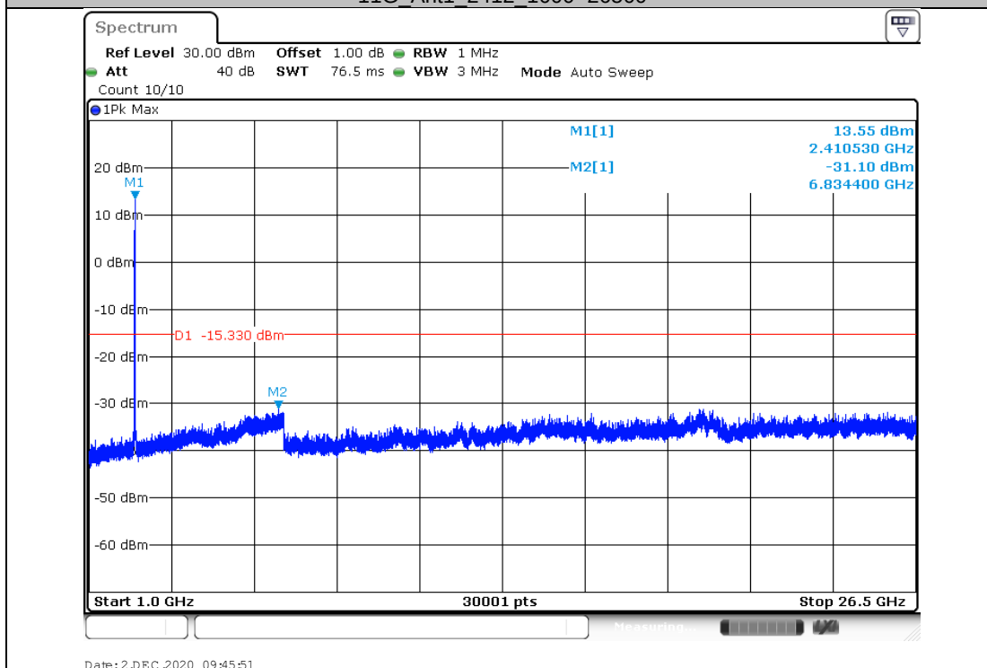
11G_Ant1_2412_1000~26500
