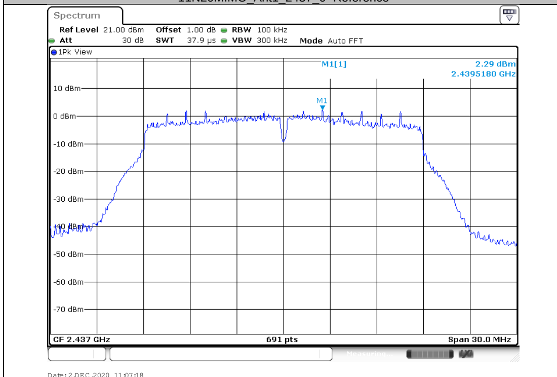
11N20MIMO_Ant1_2437_0~Reference
