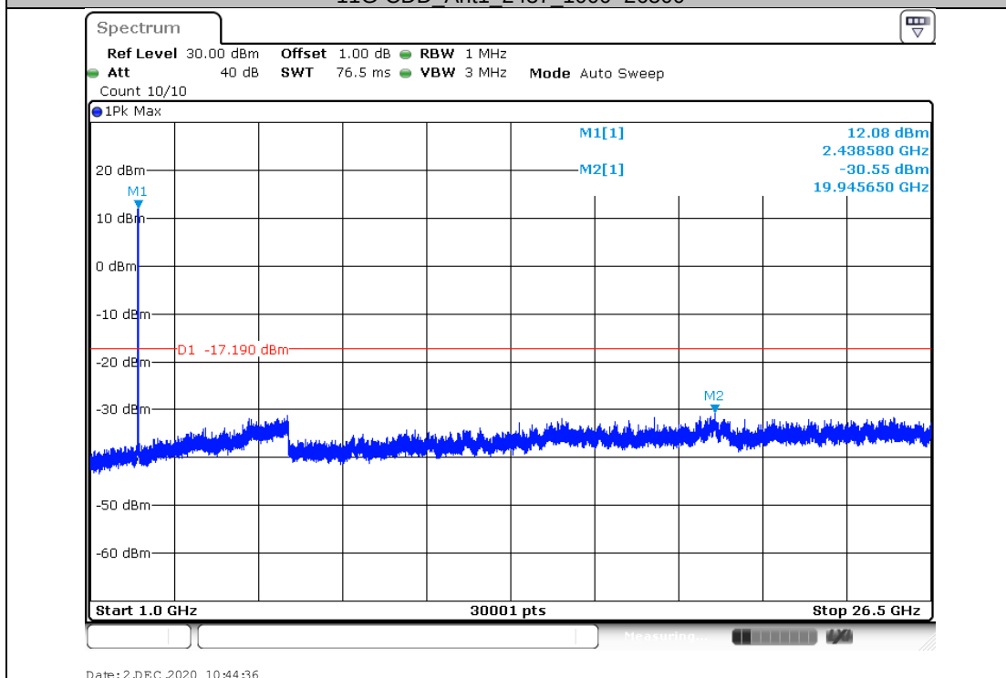
11G-CDD_Ant1_2437_1000~26500
