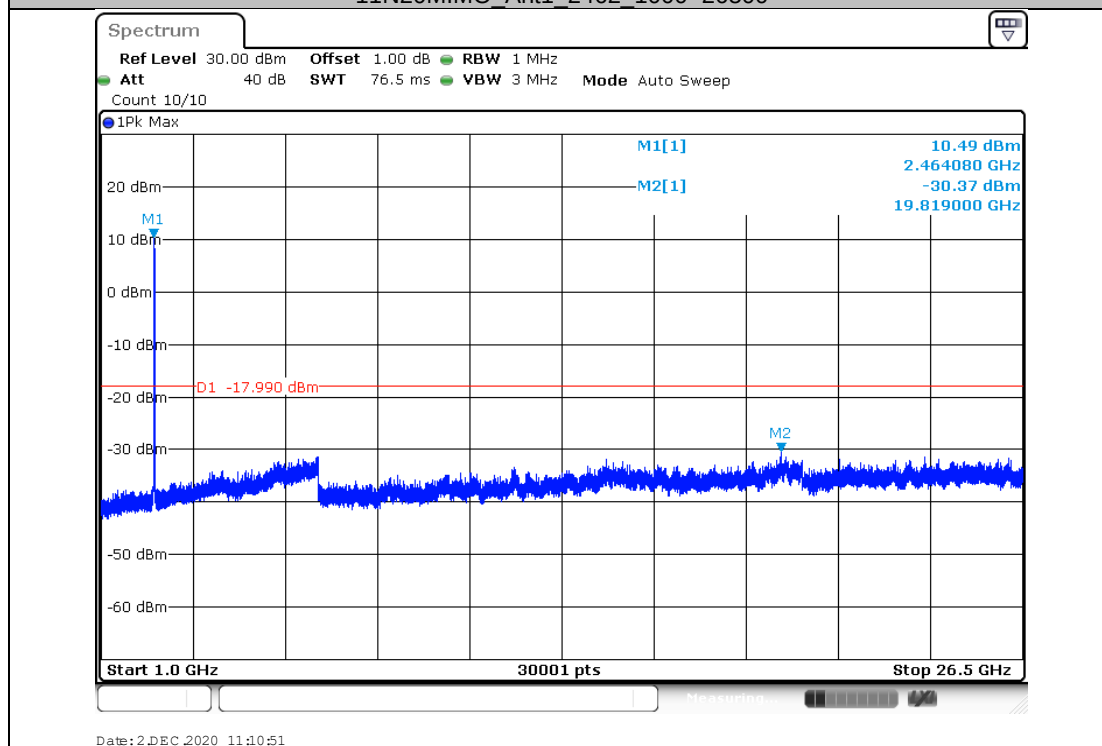
11N20MIMO_Ant1_2462_1000~26500
