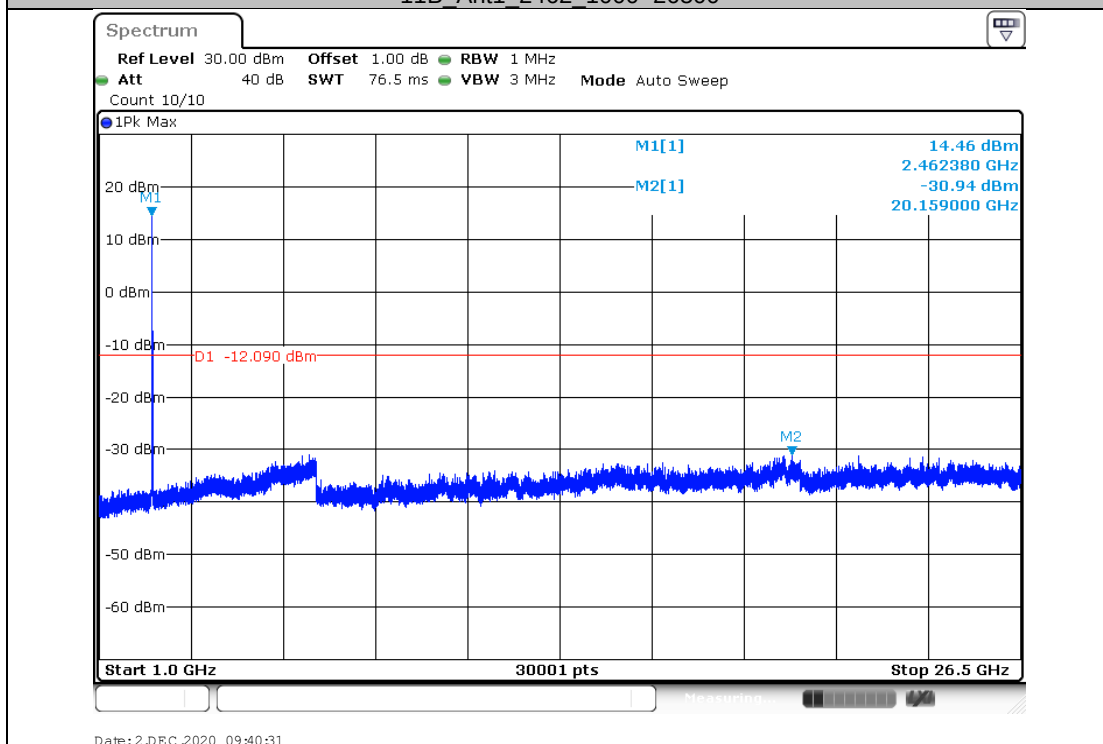
11B_Ant1_2462_1000~26500
