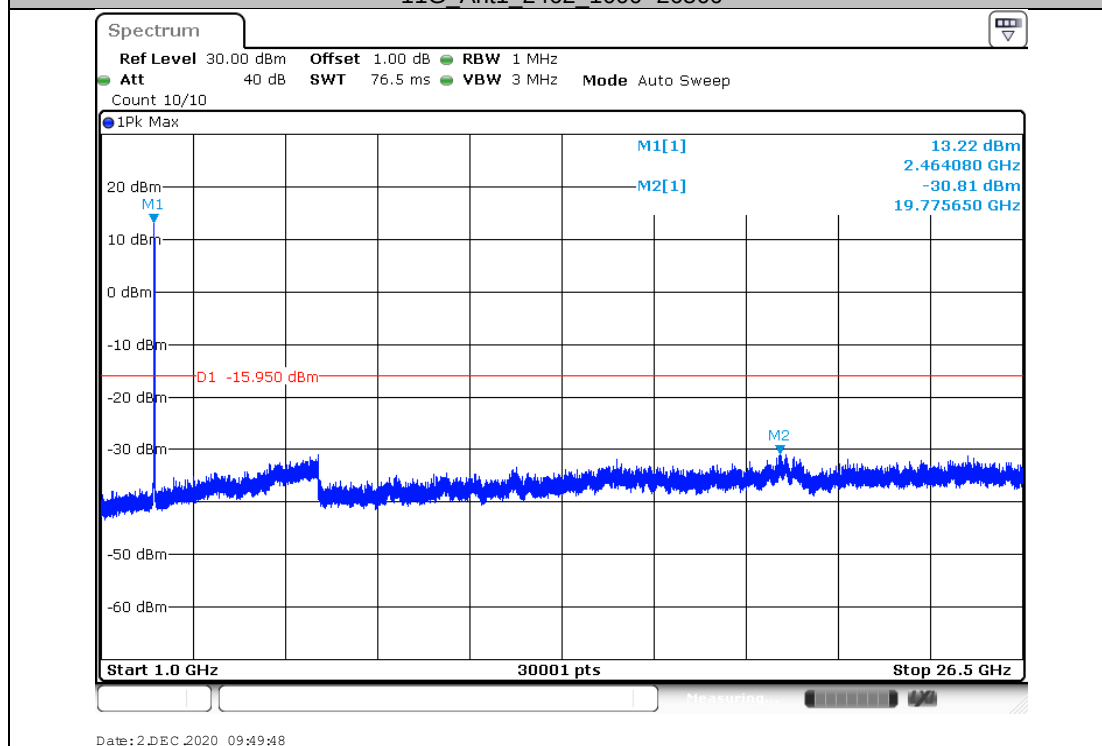
11G_Ant1_2462_1000~26500
