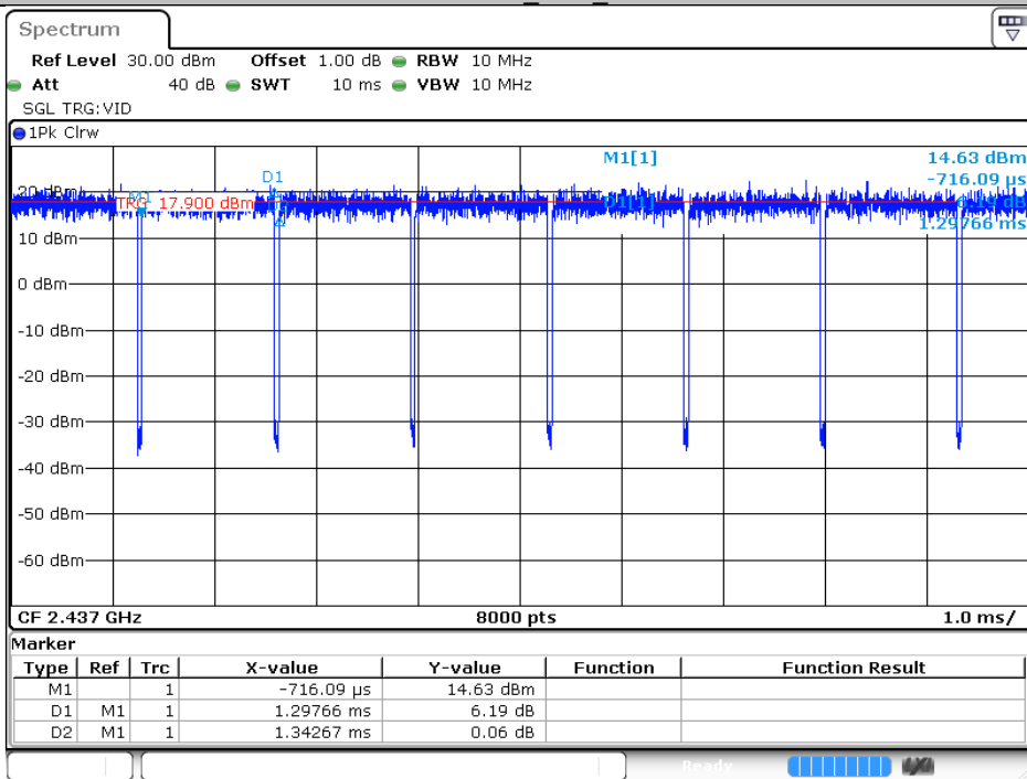
11N20MIMO_Ant1_2437
