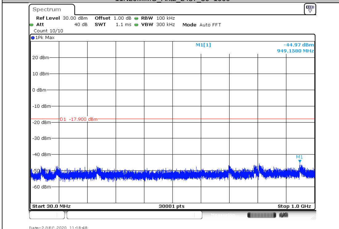
11N20MIMO_Ant2_2437_30~1000
