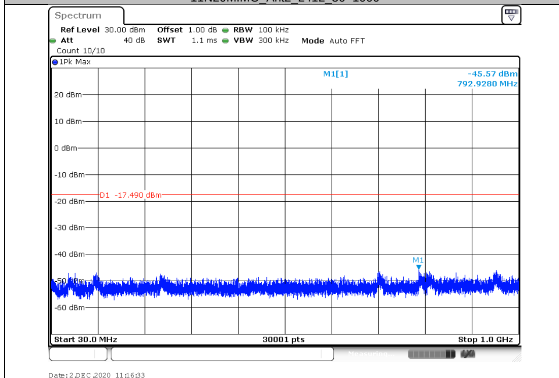
11N20MIMO_Ant2_2412_30~1000
