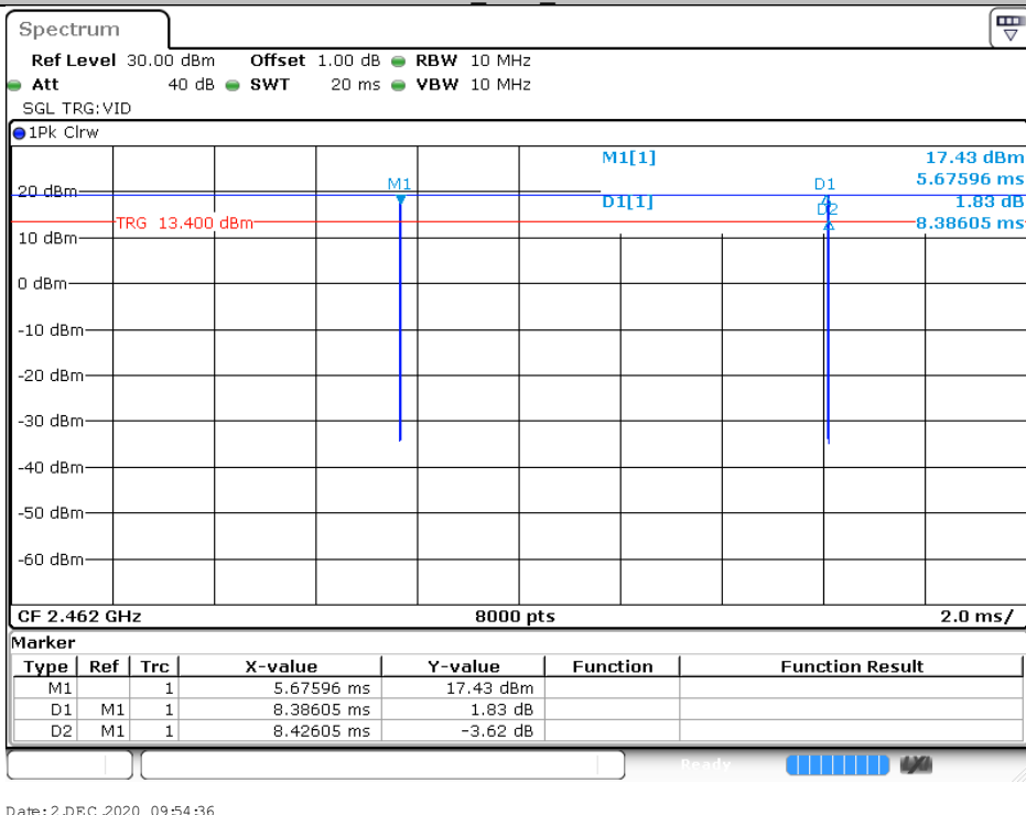
11B_Ant1_2462
