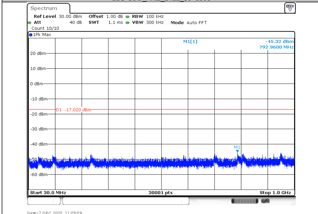
11G-CDD_Ant2_2412_30~1000
