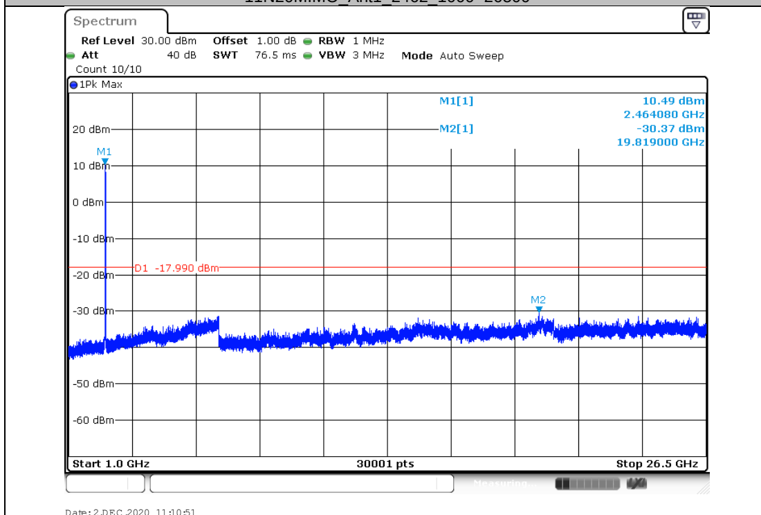
11N20MIMO_Ant1_2462_1000~26500
