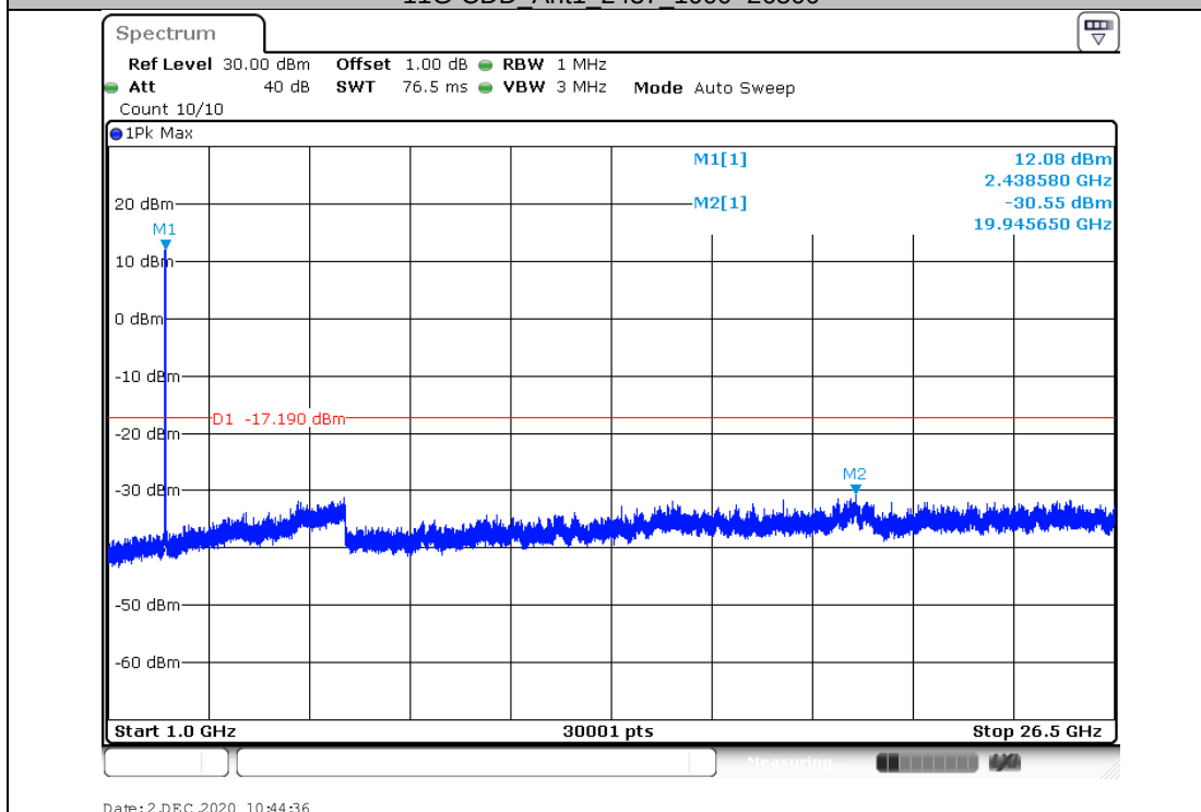
11G-CDD_Ant1_2437_1000~26500
