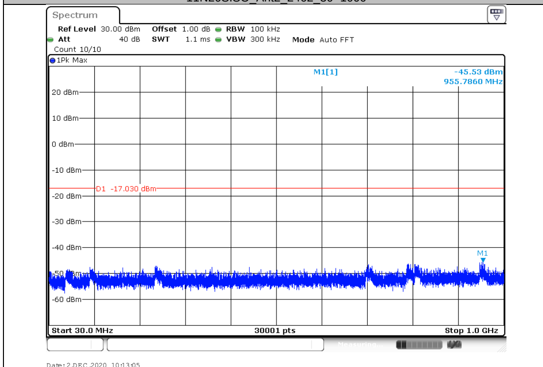
11N20SISO_Ant2_2462_30~1000
