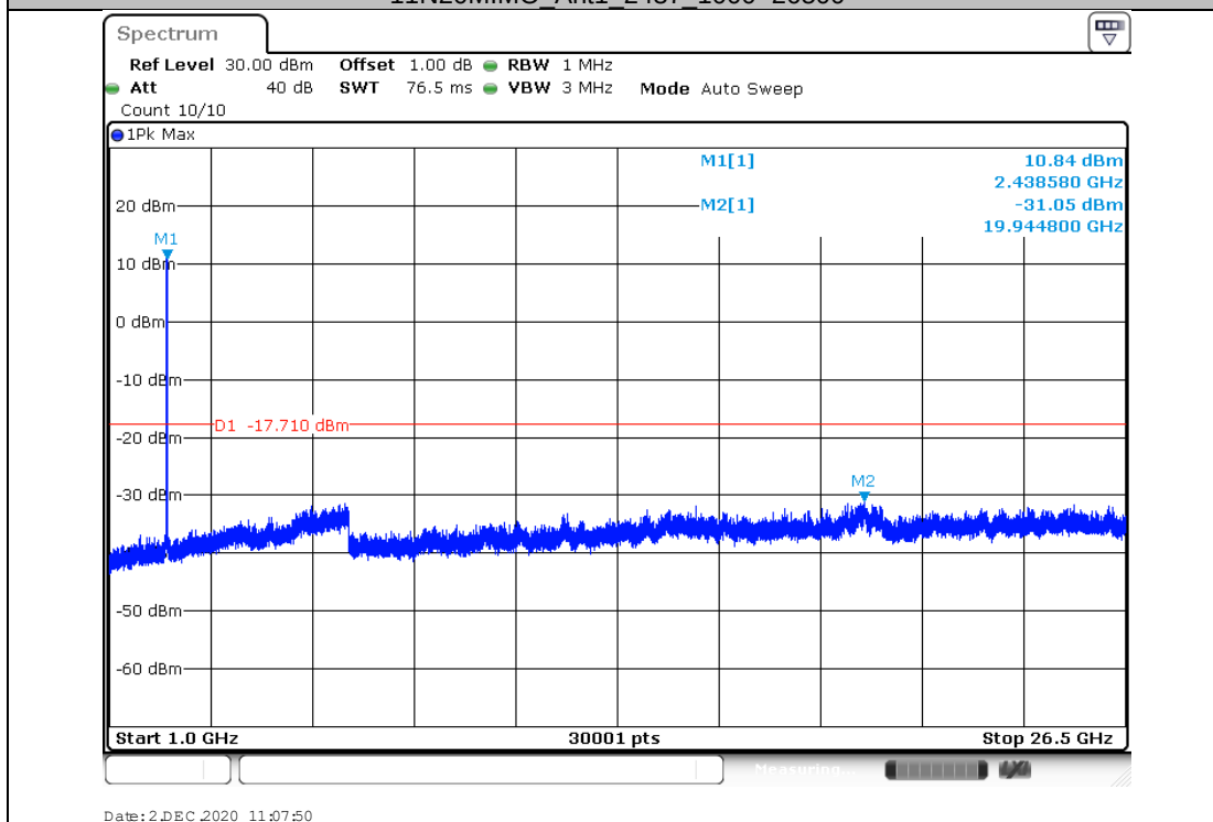
11N20MIMO_Ant1_2437_1000~26500
