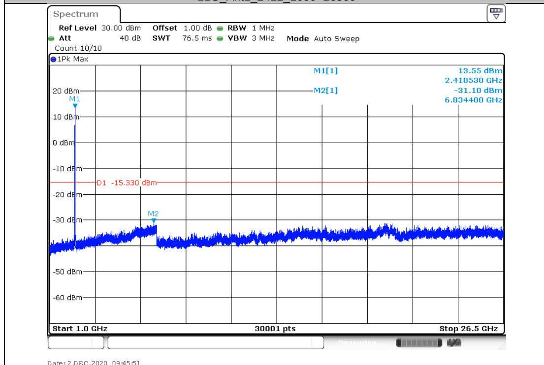
11G_Ant1_2412_1000~26500
