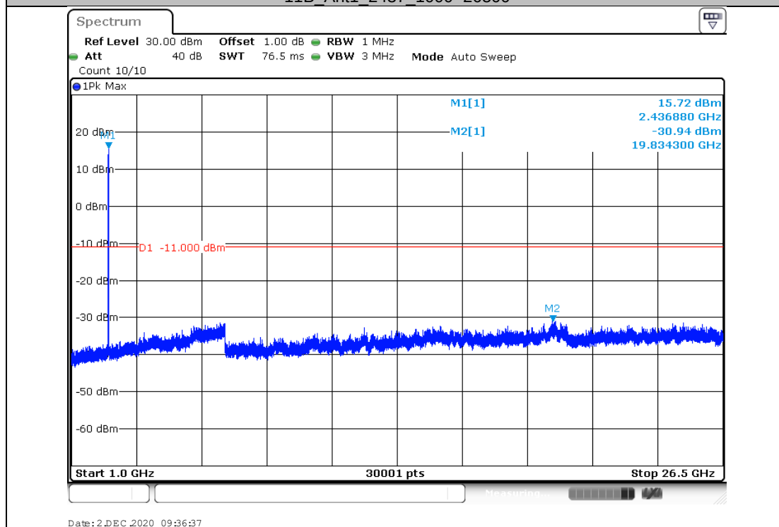
11B_Ant1_2437_1000~26500
