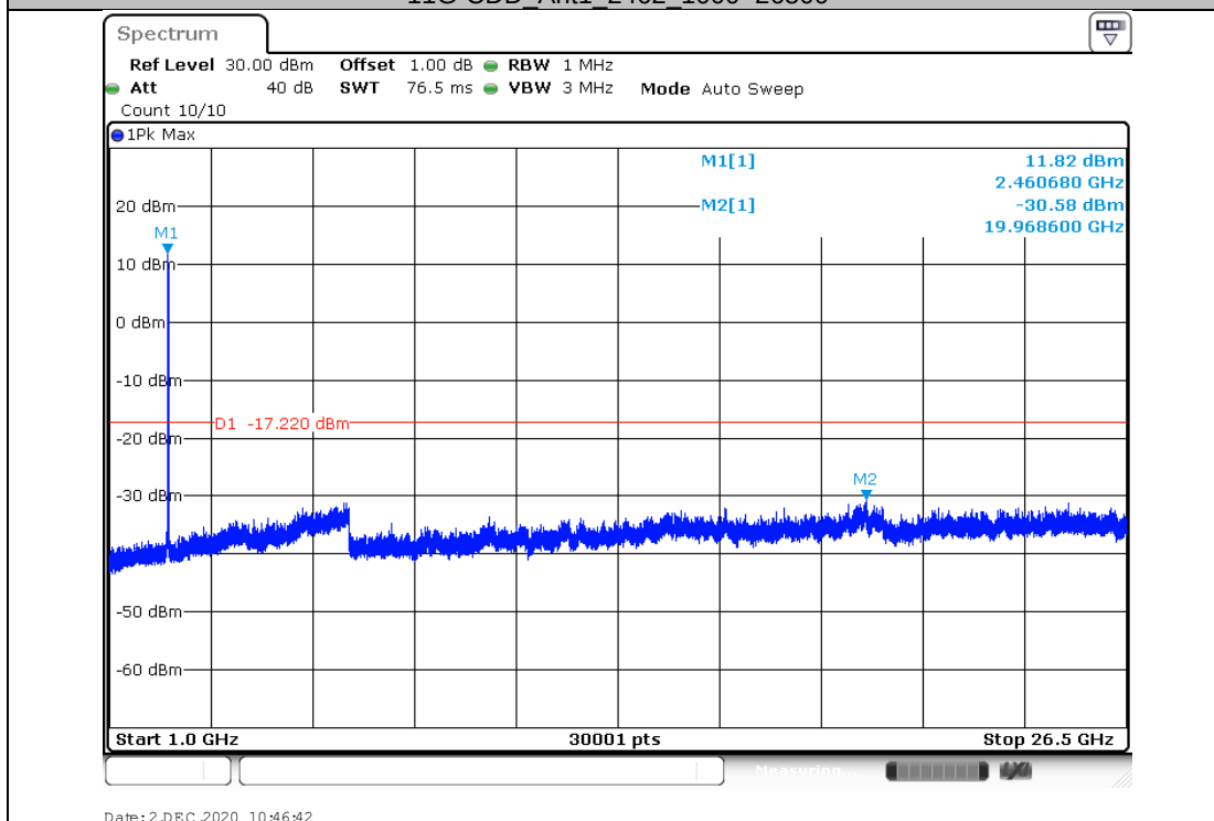
11G-CDD_Ant1_2462_1000~26500
