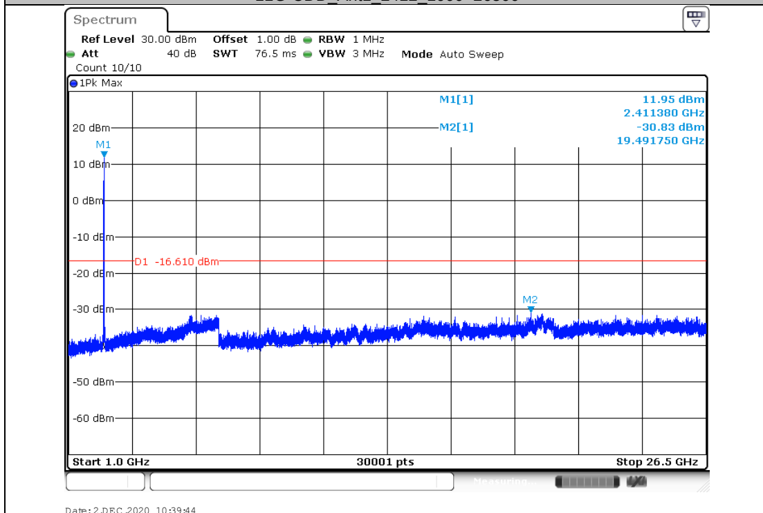
11G-CDD_Ant1_2412_1000~26500
