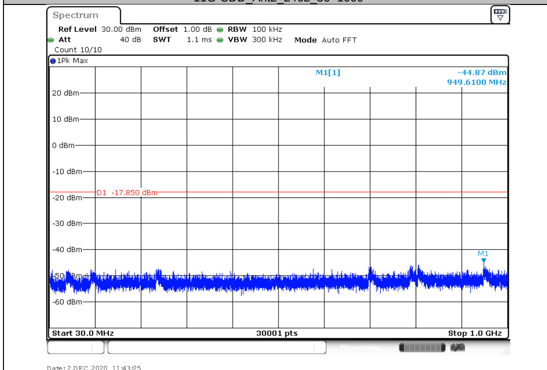
11G-CDD_Ant2_2462_30~1000
