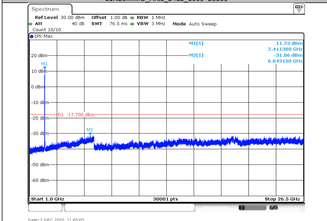
11N20MIMO_Ant1_2412_1000~26500
