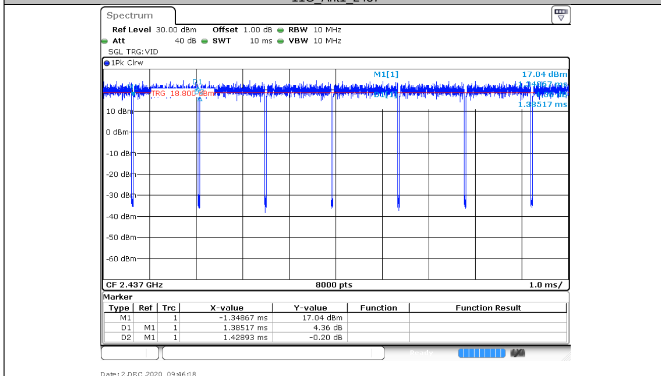
11G_Ant1_2437
