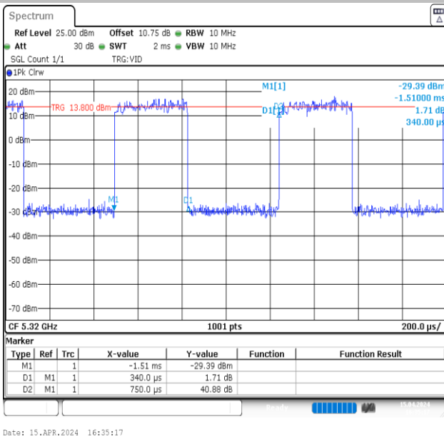
NTNV-11N20MIMO-Ant1-5320
