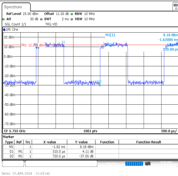
NTNV-11N40MIMO-Ant1-5755
