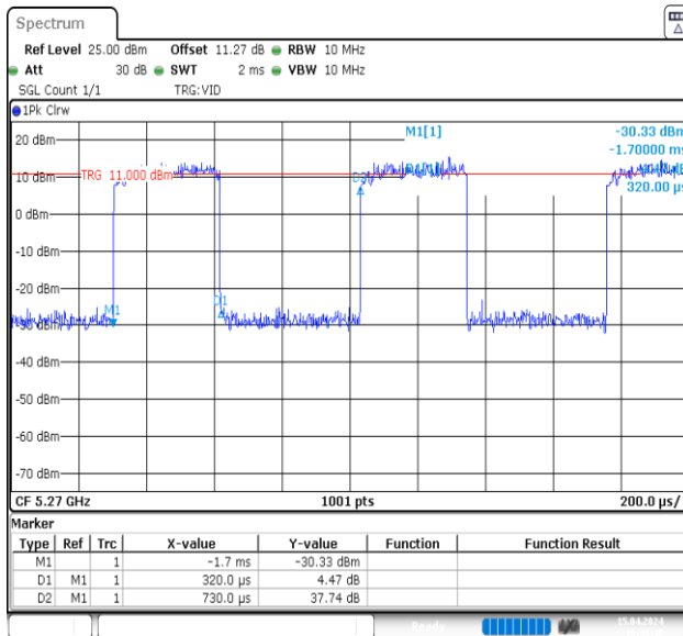
NTNV-11N40MIMO-Ant1-5270
