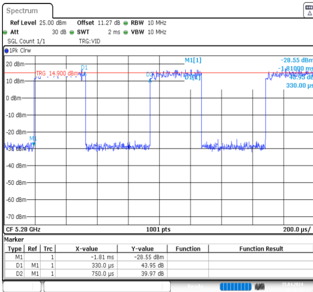
NTNV-11N20MIMO-Ant1-5280
