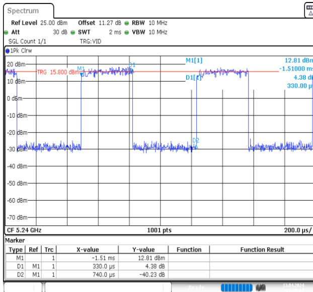
NTNV-11N20MIMO-Ant1-5240
