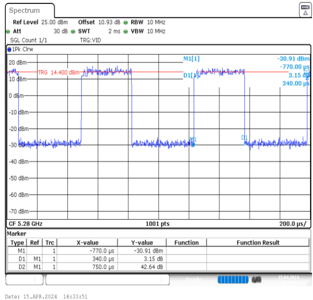
NTNV-11N20MIMO-Ant2-5280
