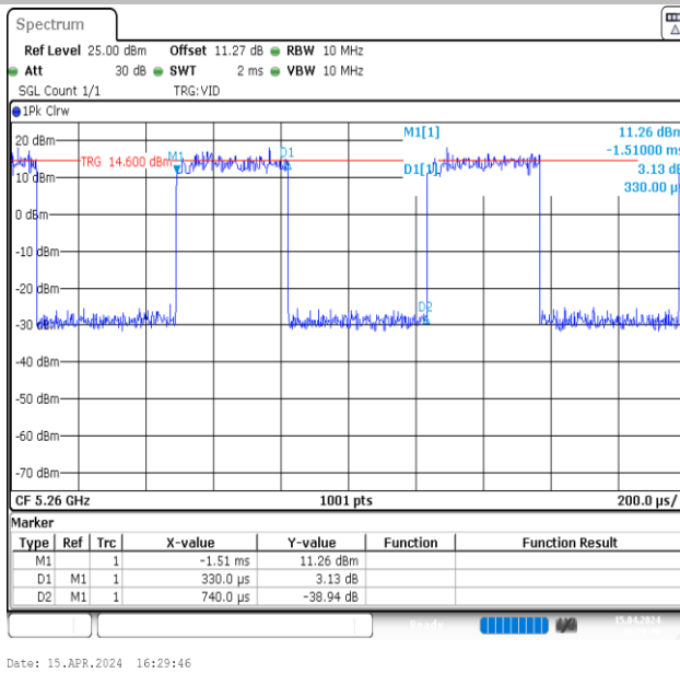
NTNV-11N20MIMO-Ant1-5260
