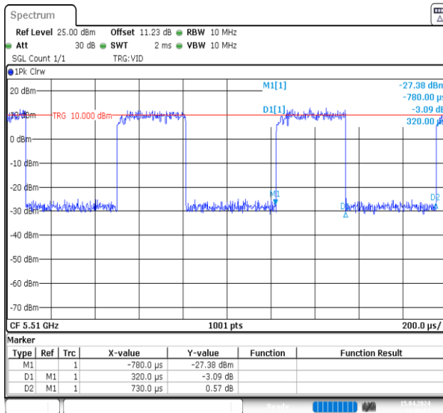
NTNV-11N40MIMO-Ant1-5510
