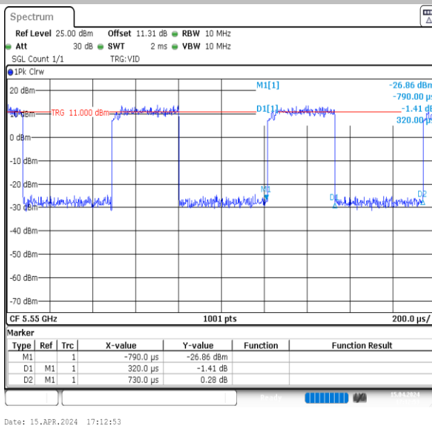
NTNV-11N40MIMO-Ant1-5550
