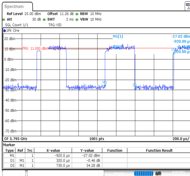
NTNV-11N40MIMO-Ant1-5795
