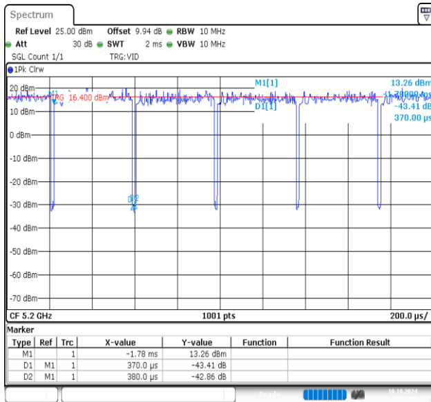
NTNV-11AC20MIMO-Ant1-5200
