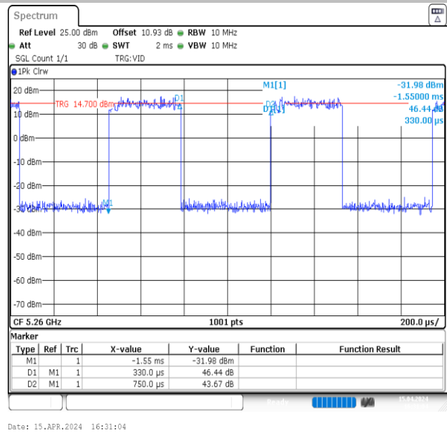
NTNV-11N20MIMO-Ant2-5260
