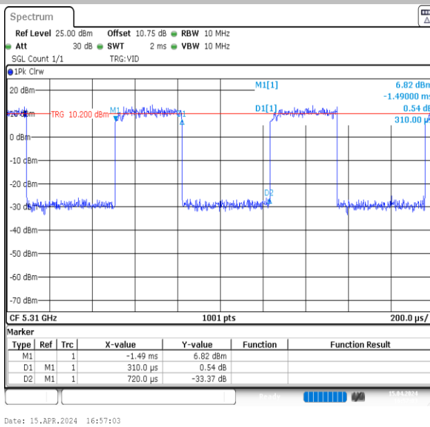
NTNV-11N40MIMO-Ant1-5310
