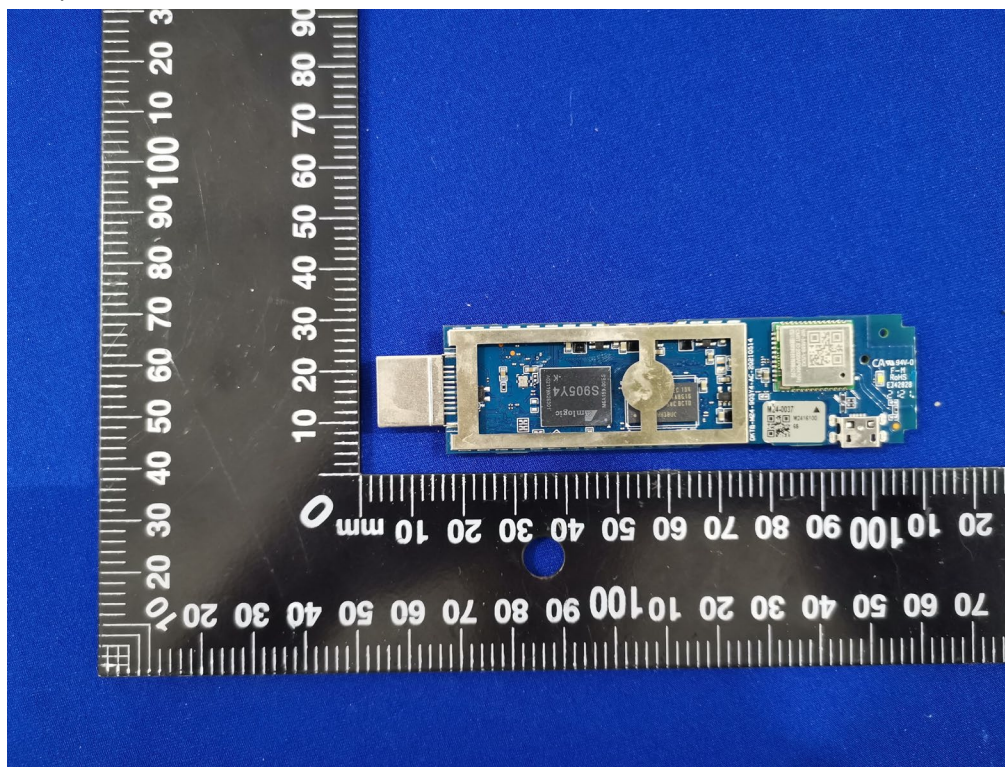
2)EUT Photo
