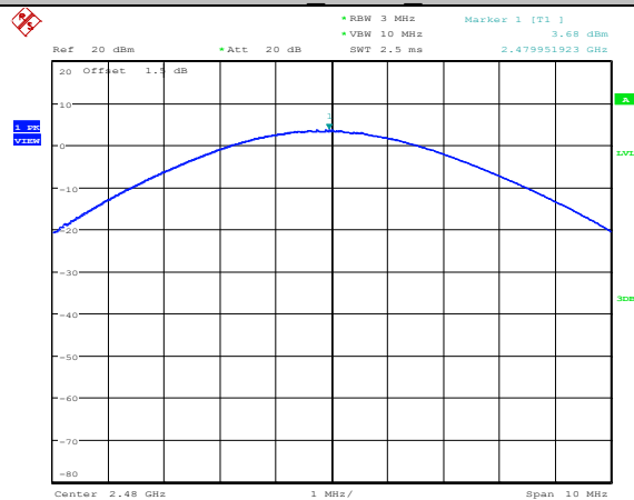
DH5_ANT1_2480
