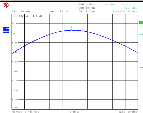
DH5_ANT1_2441
