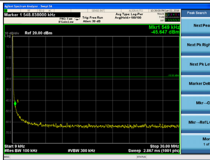
9KHz~30MHz
