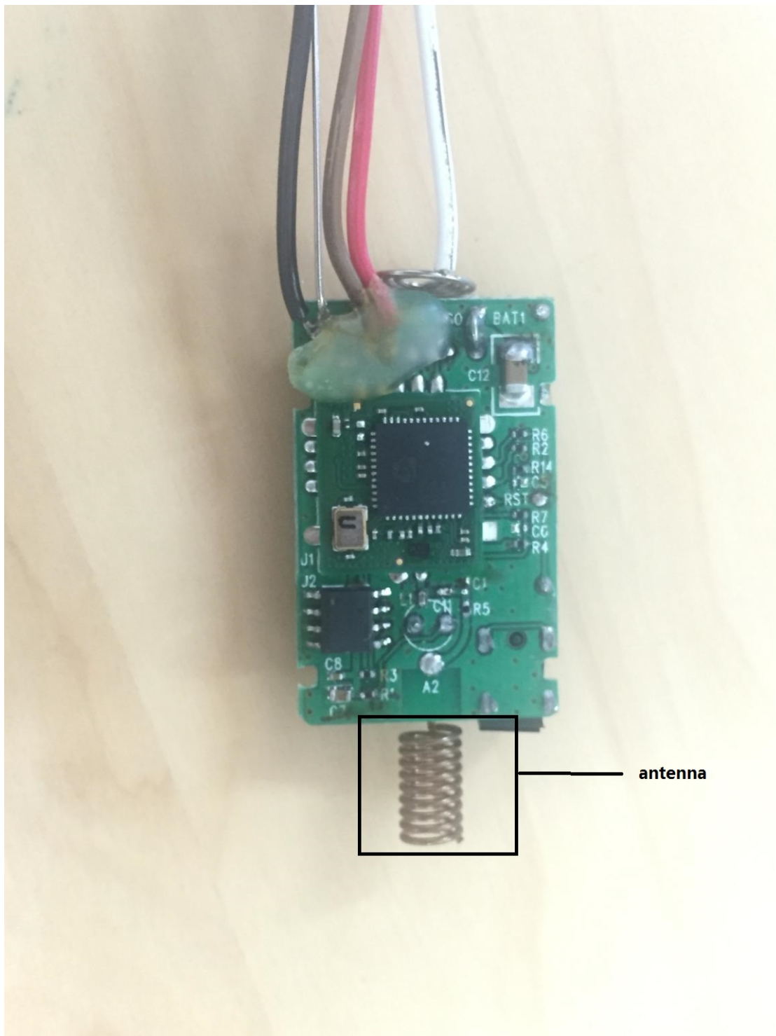
EUT
