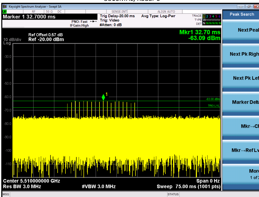
5510MHz, Radar 0
