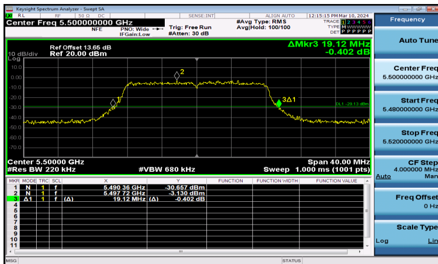
11A-Ant1-5500
