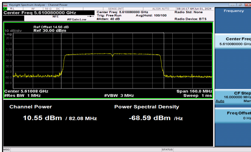
11AC80SISO-Ant1-5610-PASS
