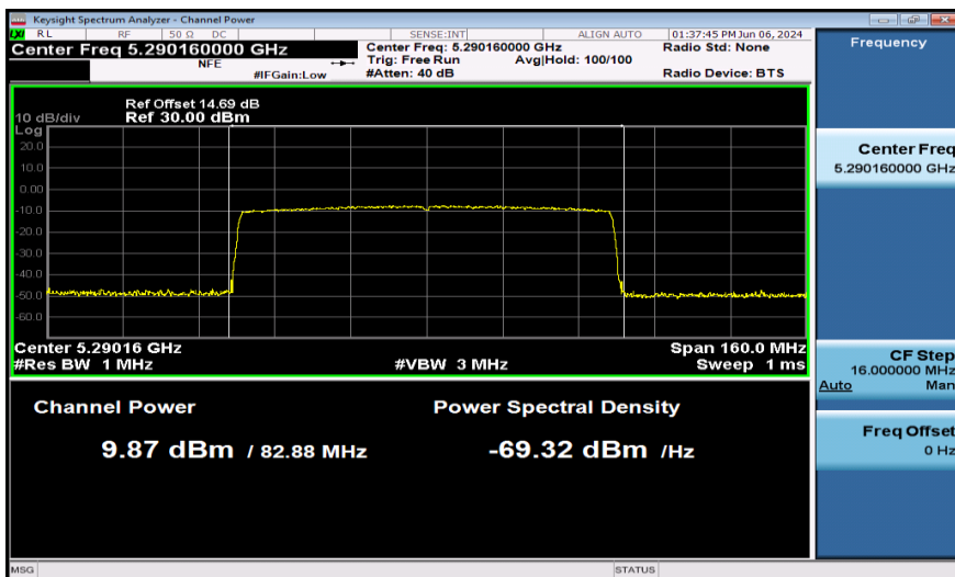
11AX80SISO-Ant1-5290-PASS
