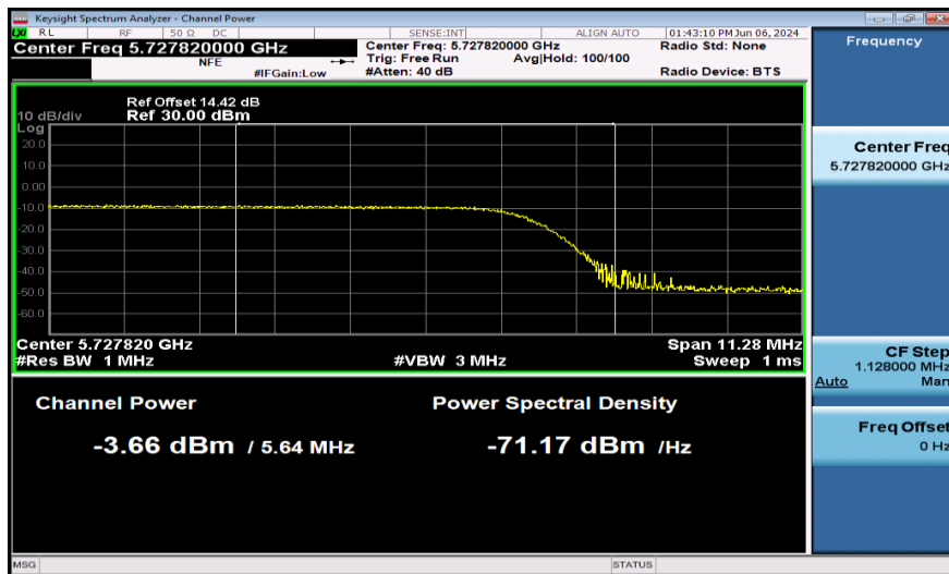
11AX80SISO-Ant1-5690_UNII-3-PASS
