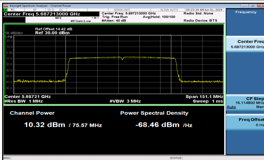
11AC80SISO-Ant1-5690_UNII-2C-PASS
