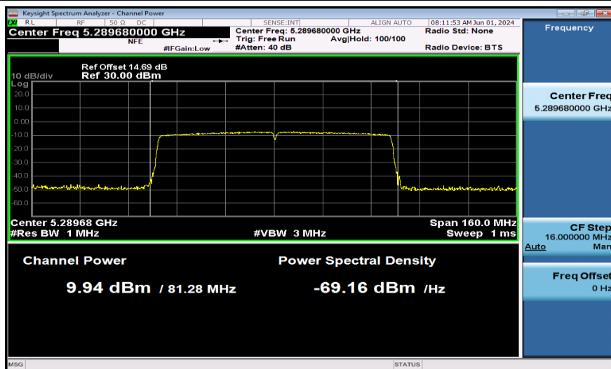
11AC80SISO-Ant1-5290-PASS
