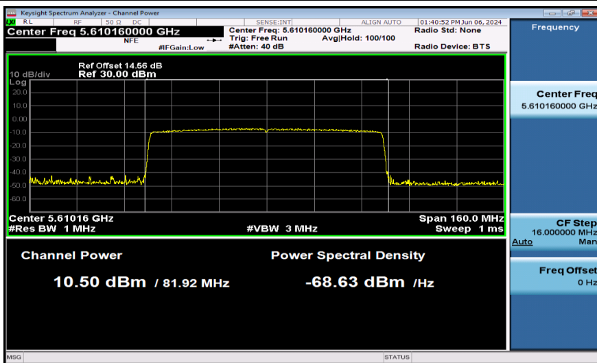
11AX80SISO-Ant1-5610-PASS
