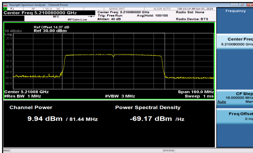
11AC80SISO-Ant1-5210-PASS
