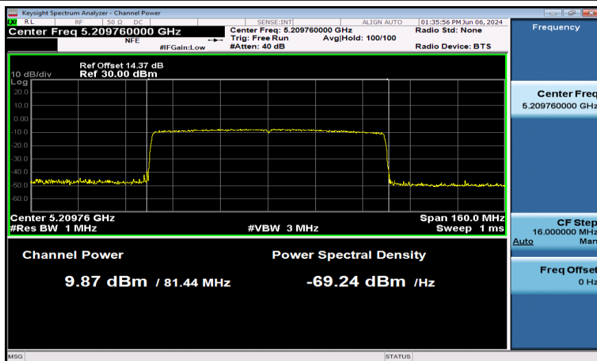
11AX80SISO-Ant1-5210-PASS
