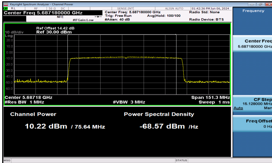
11AX80SISO-Ant1-5690_UNII-2C-PASS
