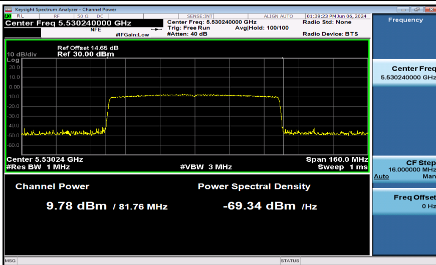
11AX80SISO-Ant1-5530-PASS
