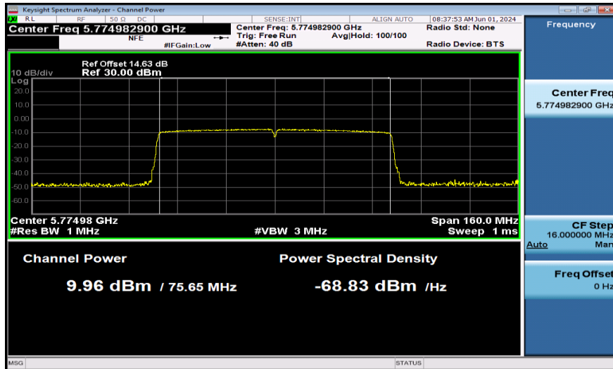
11AC80SISO-Ant1-5775-PASS
