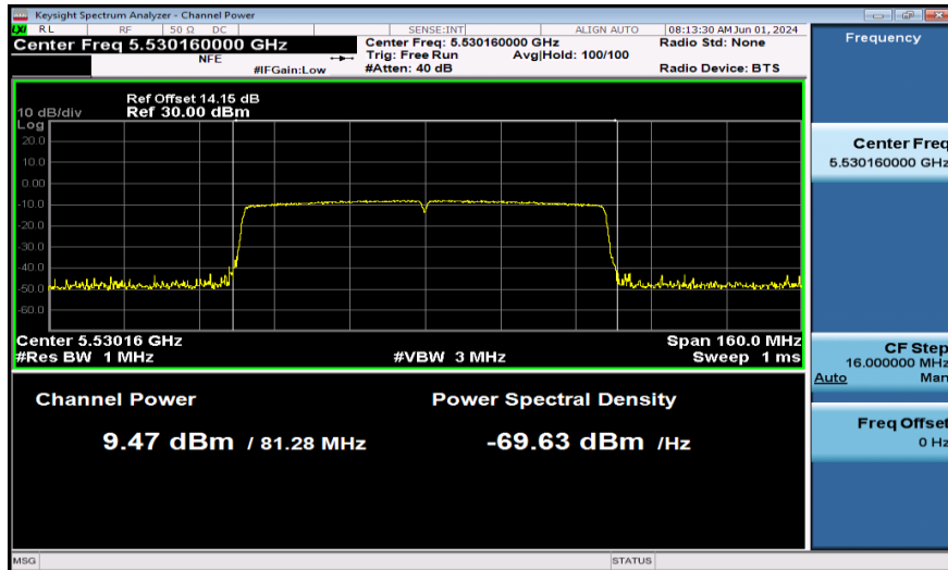
11AC80SISO-Ant1-5530-PASS
