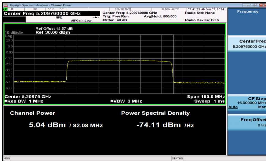
11AX80SISO-Ant1-5210-996Tone-PASS
