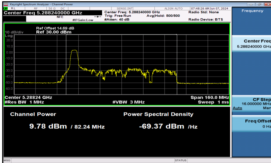
11AX80SISO-Ant1-5290-52Tone-PASS
