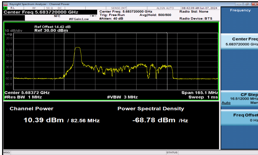
11AX80SISO-Ant1-5690_UNII-2C-52Tone-PASS
