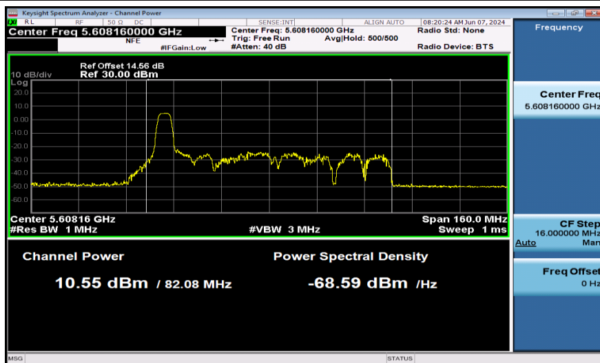
11AX80SISO-Ant1-5610-52Tone-PASS
