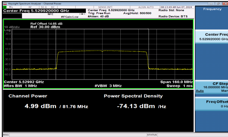
11AX80SISO-Ant1-5530-996Tone-PASS
