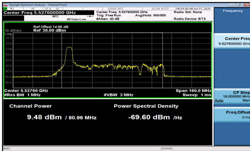
11AX80SISO-Ant1-5530-52Tone-PASS
