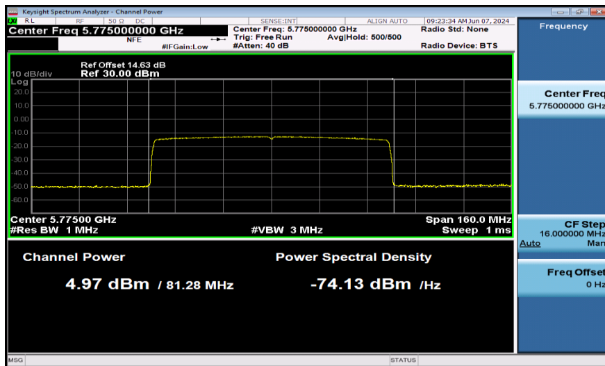
11AX80SISO-Ant1-5775-996Tone-PASS
