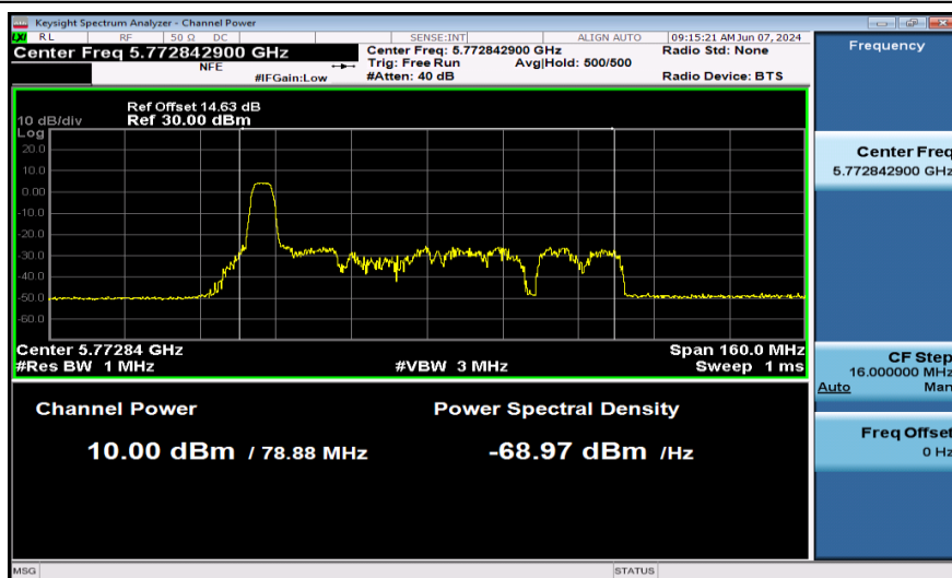
11AX80SISO-Ant1-5775-52Tone-PASS
