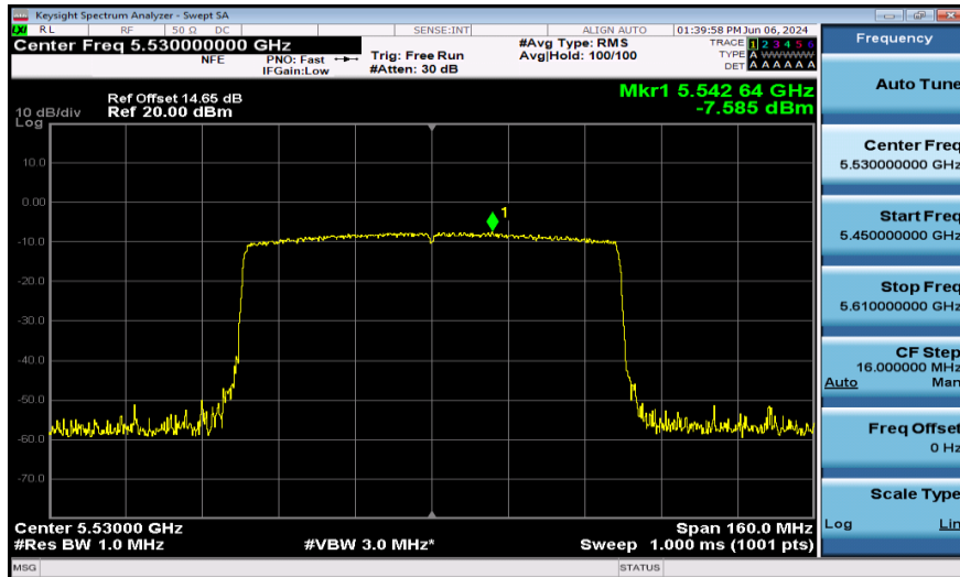
11AX80SISO-Ant1-5530-PASS
