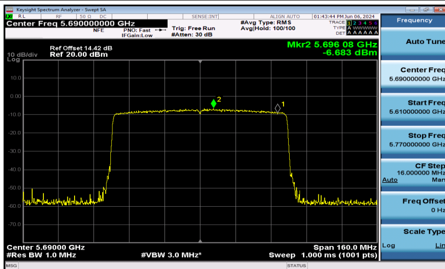
11AX80SISO-Ant1-5690_UNII-2C-PASS
