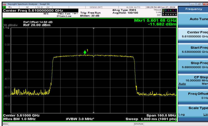
11AX80SISO-Ant1-5610-996Tone-PASS
