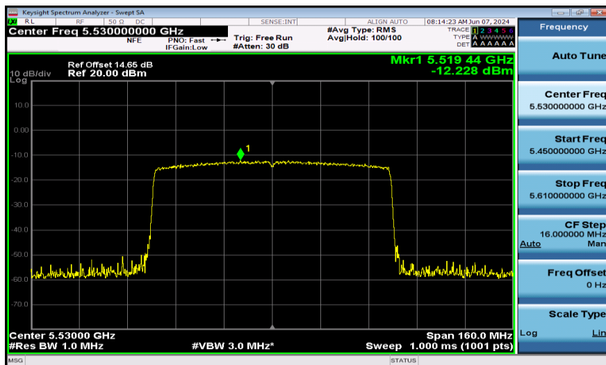
11AX80SISO-Ant1-5530-996Tone-PASS
