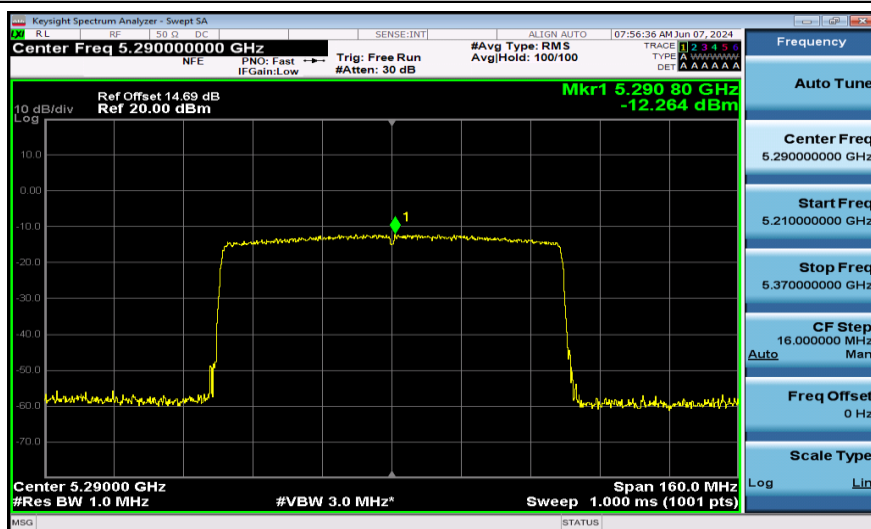
11AX80SISO-Ant1-5290-996Tone-PASS
