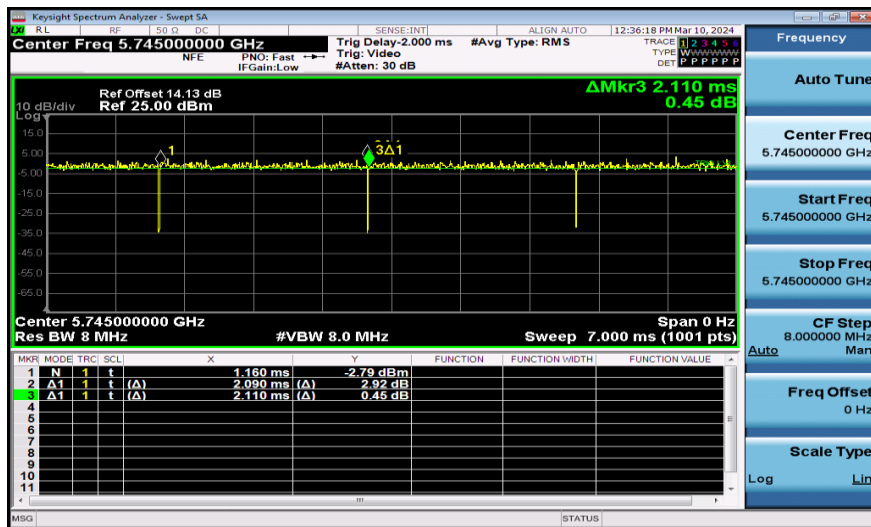
NTNV-11A-Ant1-5745
