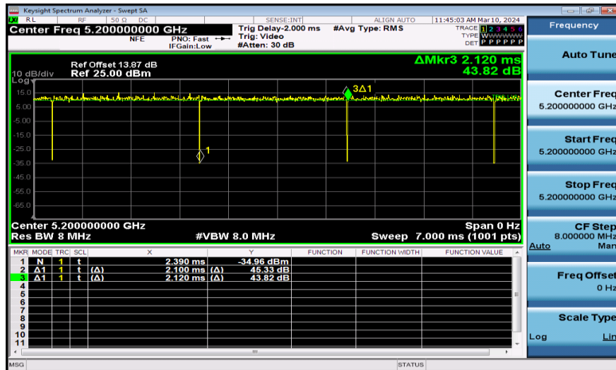
NTNV-11A-Ant1-5200
