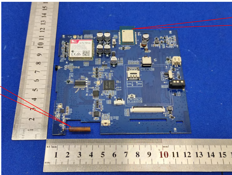
2.4GWIFI Antenna
