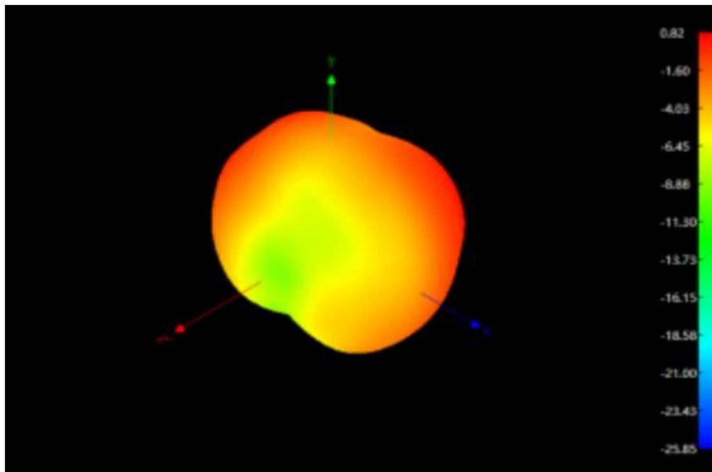
2480MHz 3D
