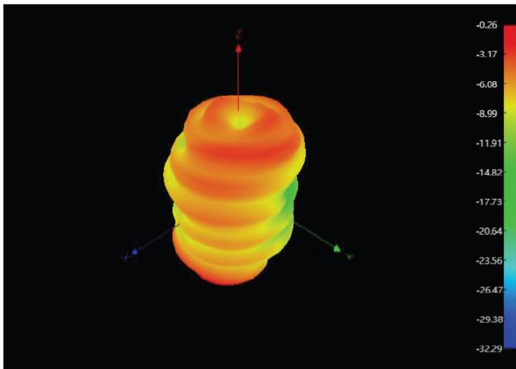
2500MHz 3D
