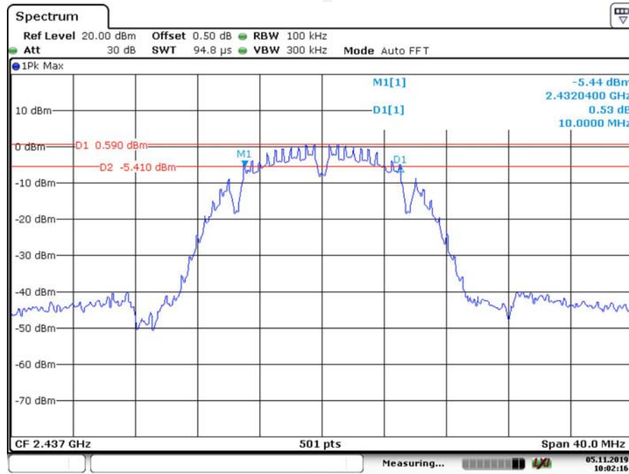
802.11 b_Middle
