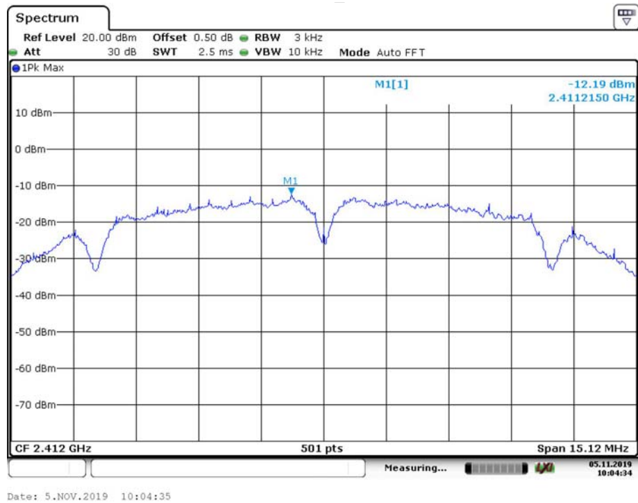
802.11 b Low
