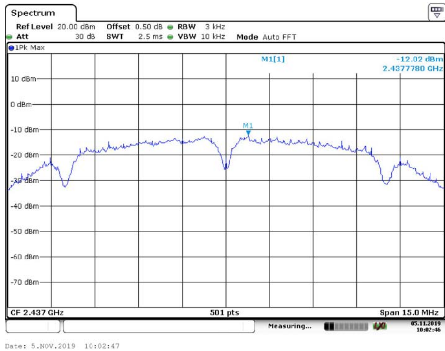
802.11 b Middle
