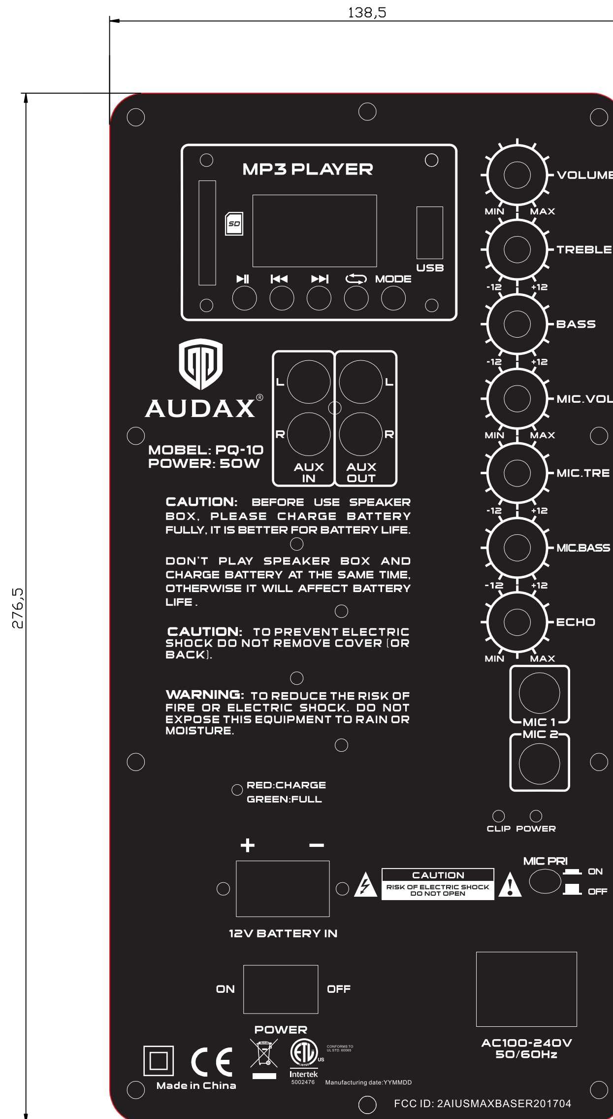
PSQ-10/PRX-10H/PRX-10PRH-10V通用面板
