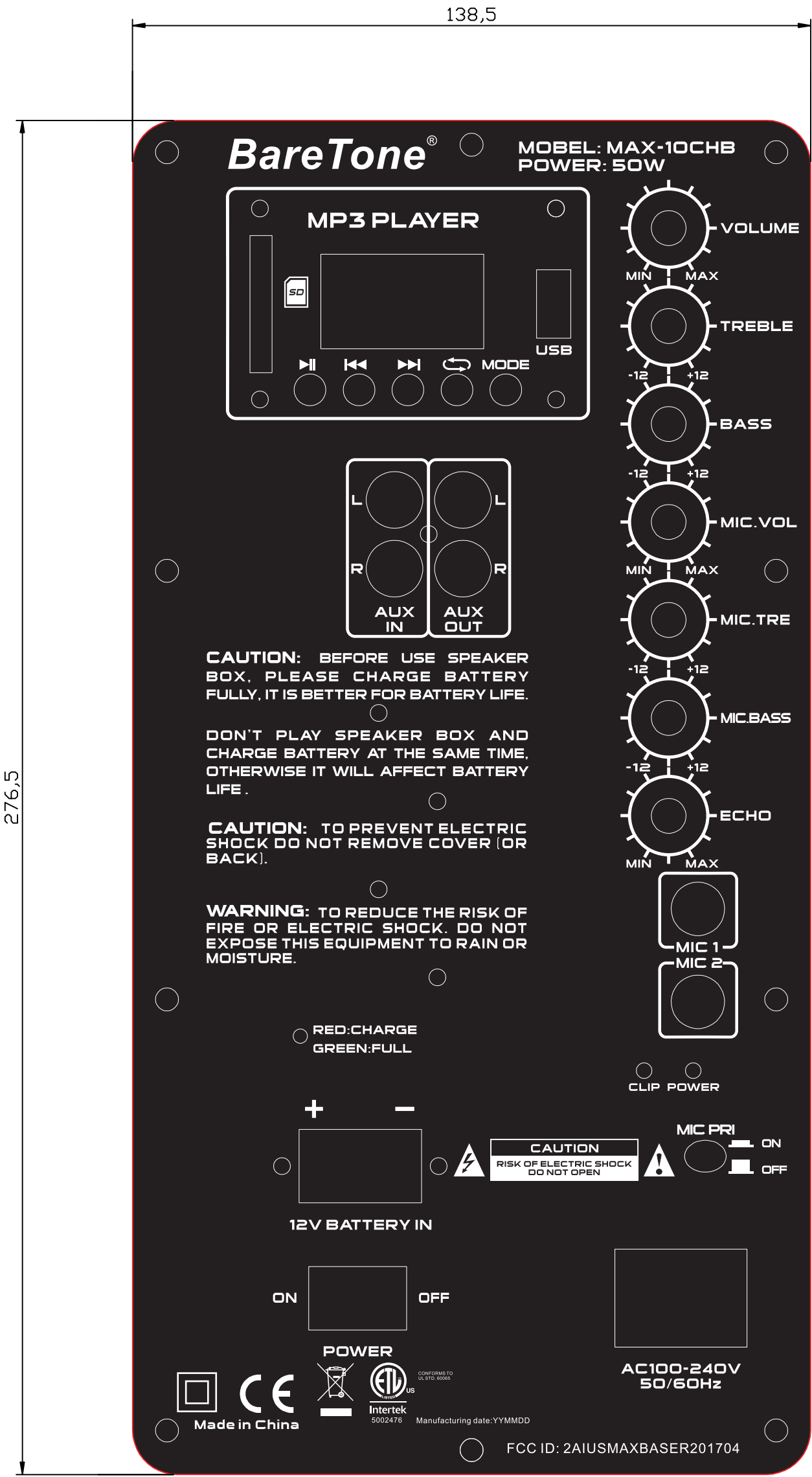
MAX-10-10MB/MAX-10CHB/MAX-10CBMAX-10RB通用面板
