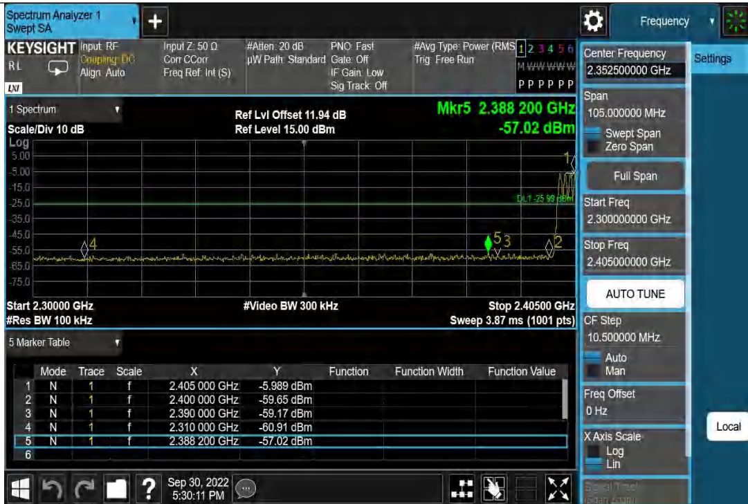
DH5_Ant1_Low_Hop_2402
