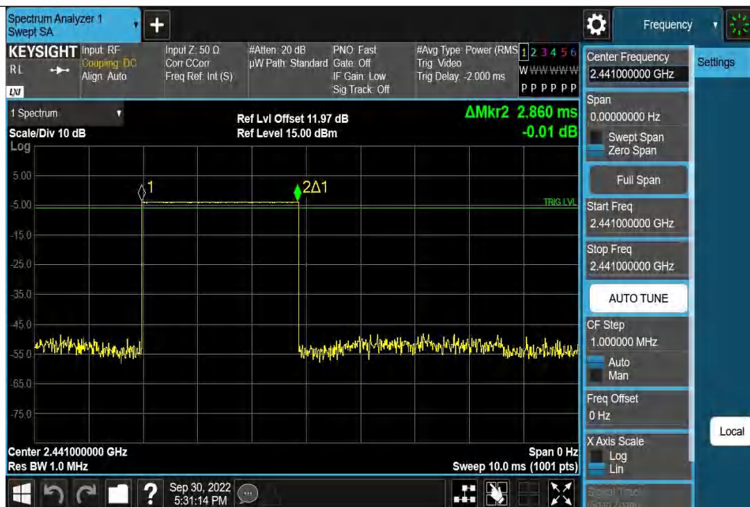
DH5_Ant1_Hop
