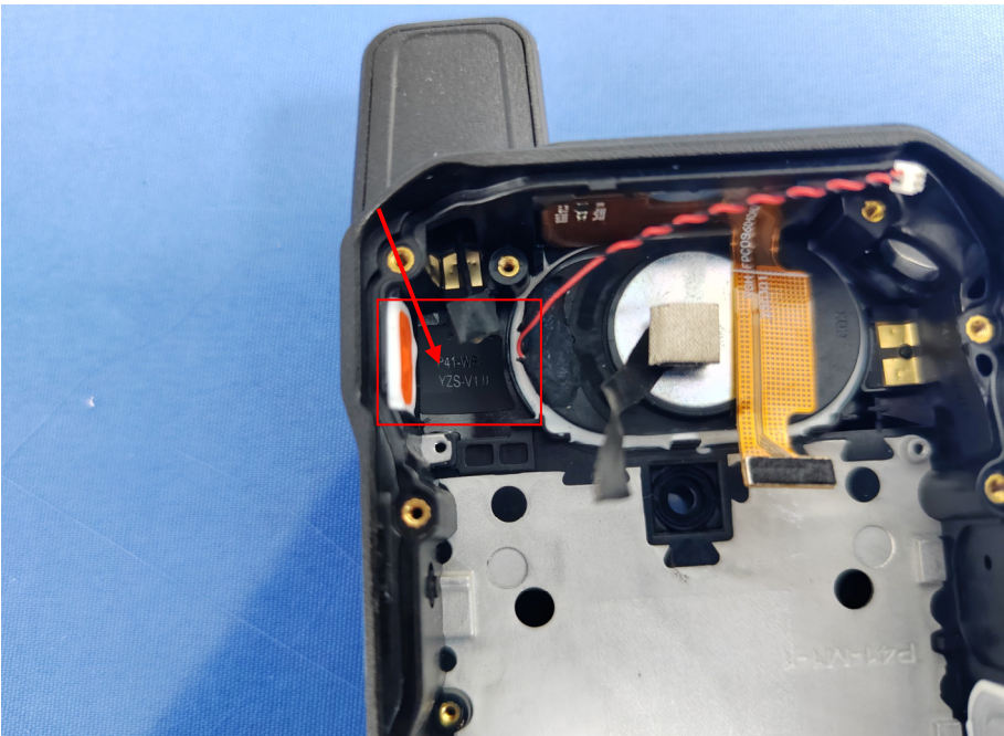
BT/BLE/WIFI Antenna
