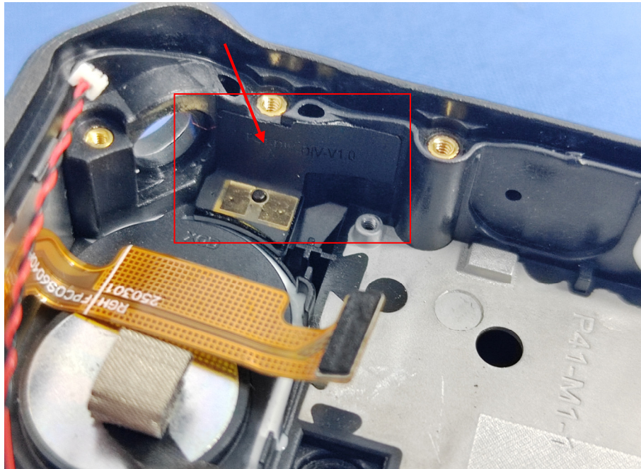
GSM/WCDMA/LTE DIV Antenna
