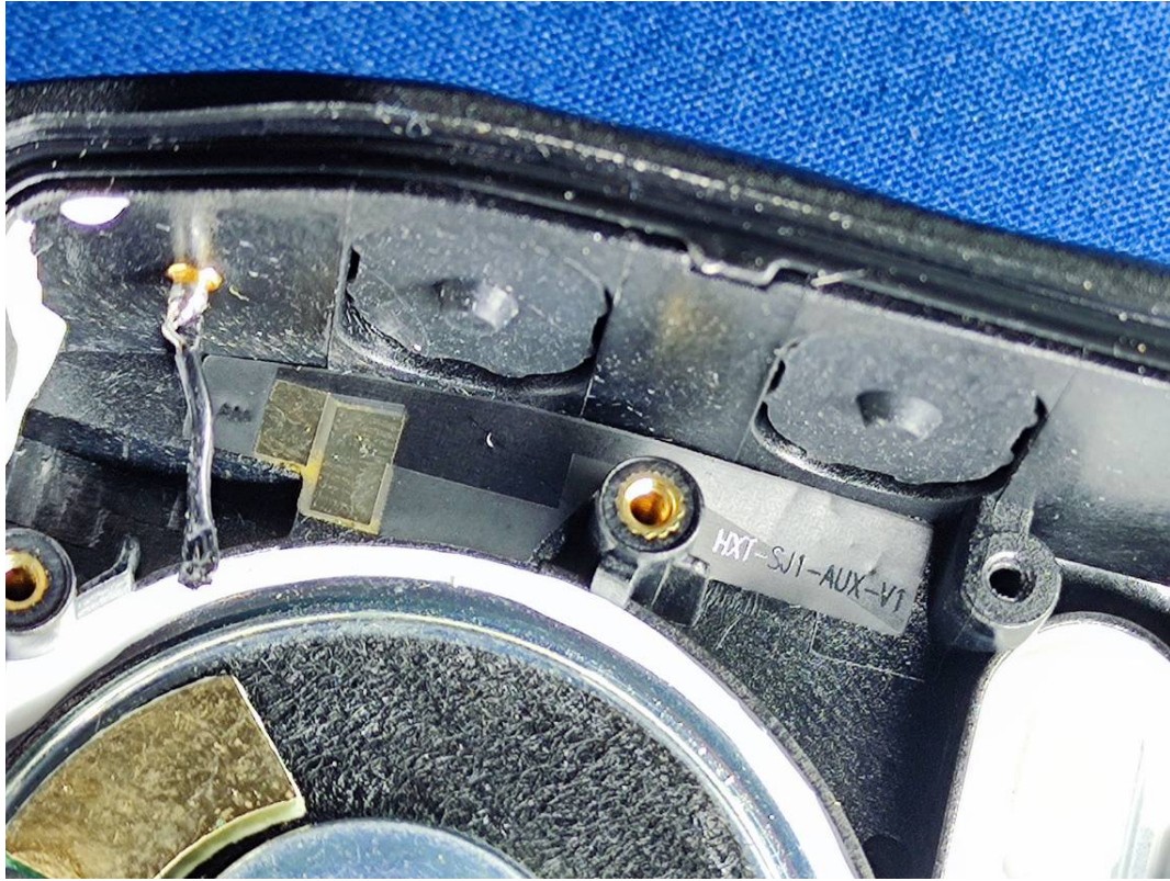
Bluetooth&WIFI Antenna
