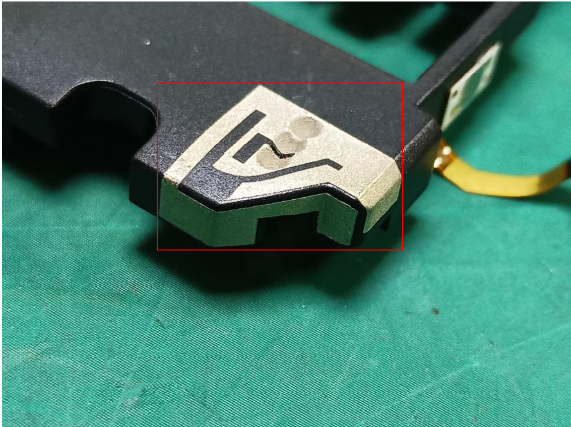
BT/Wi-Fi/GPS ANT
