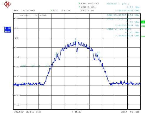
802.11b_2442MHz
