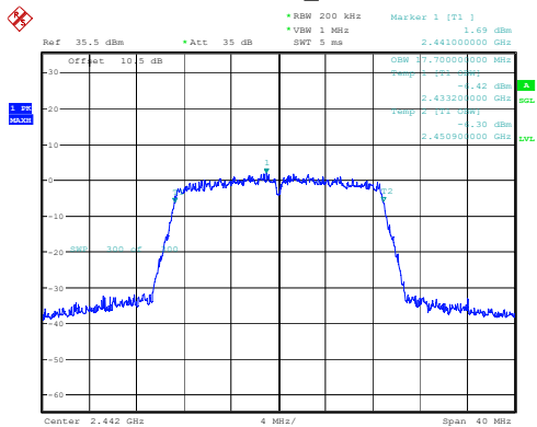
802.11n20_2442MHz
