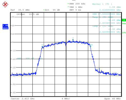
802.11n20_2412MHz
