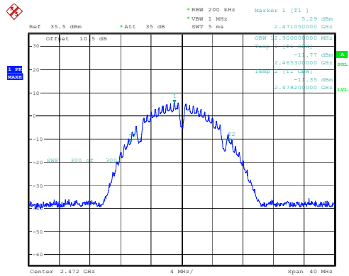
802.11b_2472MHz
