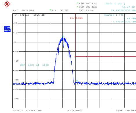
802.11b_2472MHz
