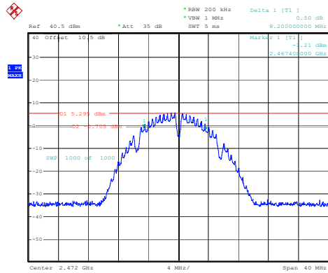
802.11b_2472MHz
