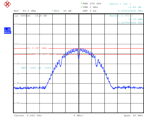
802.11b_2442MHz
