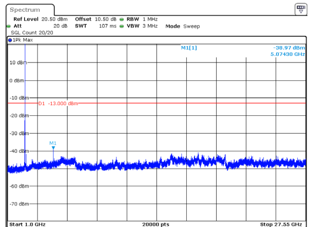
5MHz_Low_QPSK_25@0(1GHz~27.55GHz)
