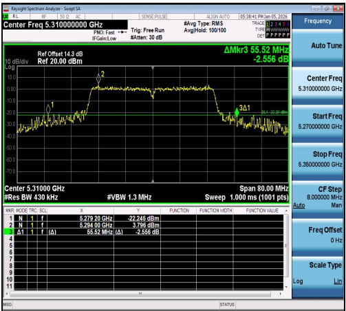
11N40SISO-Ant1-5310
