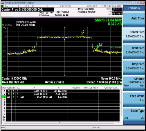
11AC80SISO-Ant1-5530
