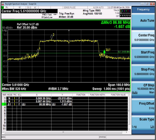
11AC80SISO-Ant1-5610
