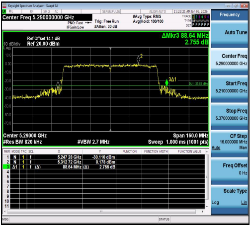
11AC80SISO-Ant1-5290
