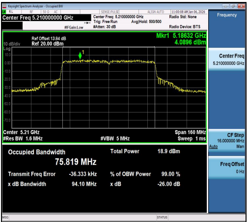
11AC80SISO-Ant1-5210
