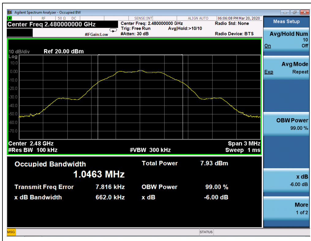
(Channel 39, 2480MHz)
