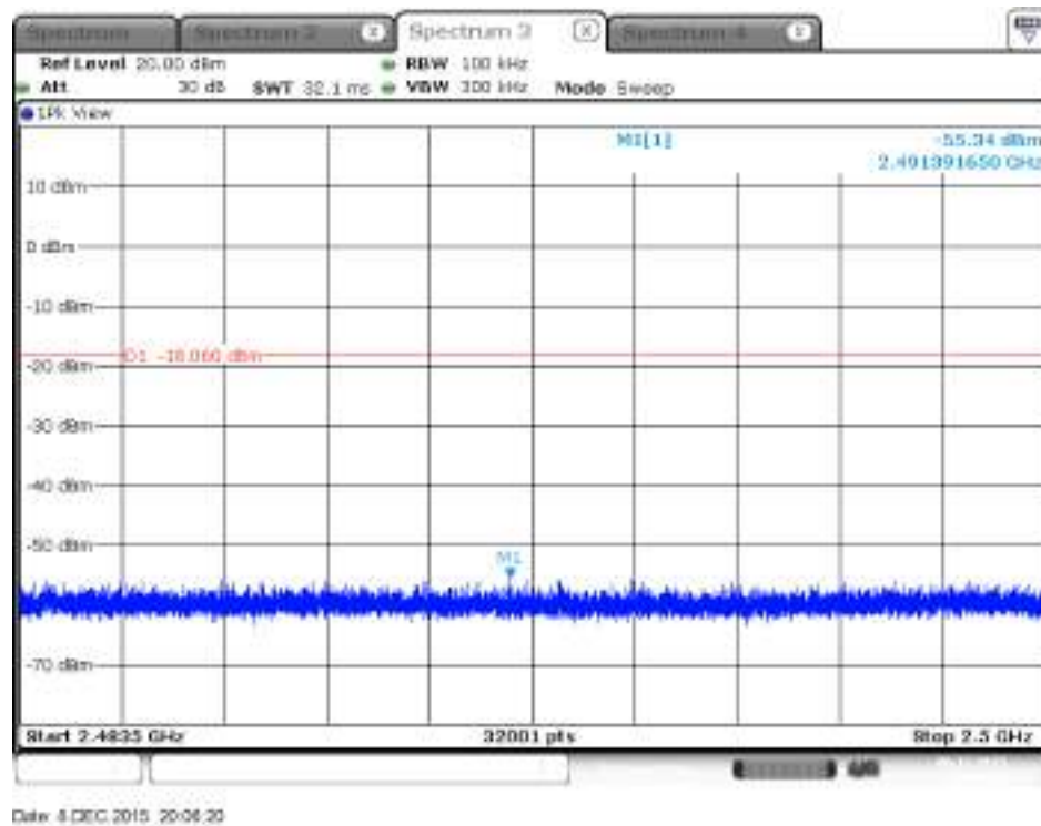
Plot on Configuration IEEE 802.11b / 2412 MHz / 2483.5MHz~2500MHz (down 30dBc) / Chain 2
