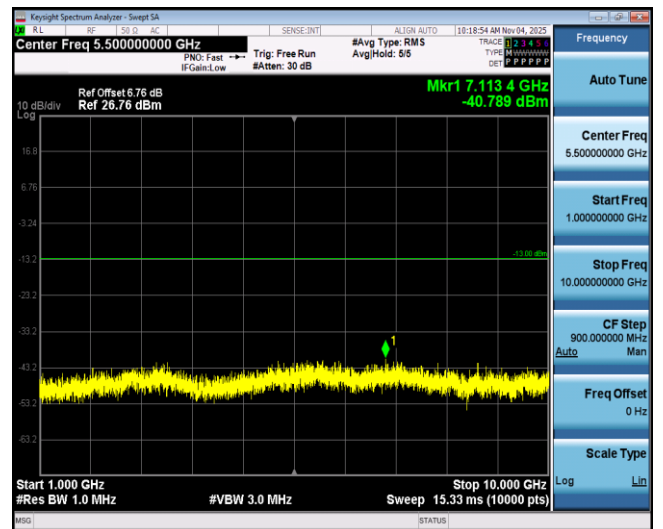
Band5-10MHz-QPSK-20525-1RB#0-Range2:1000~1 0000MHz
