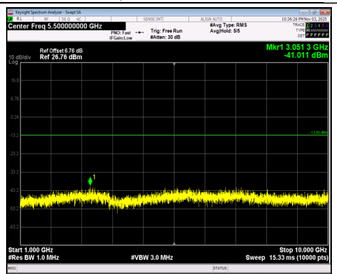
Band5-1.4MHz-QPSK-20525-1RB#0-Range2:1000~1 0000MHz
