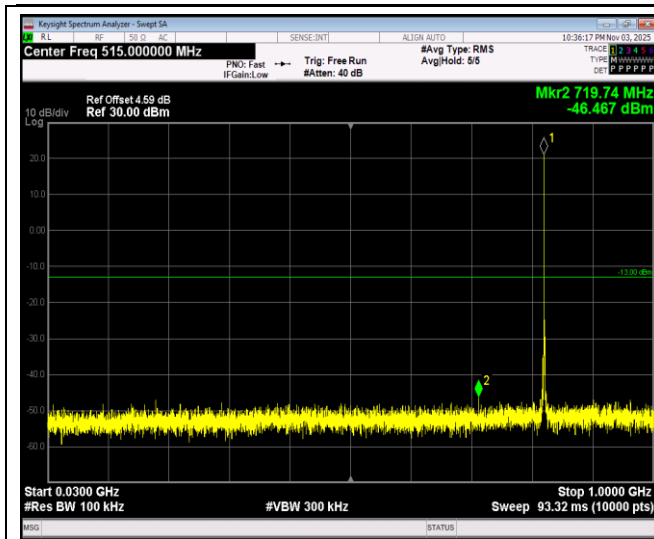
Band5-1.4MHz-QPSK-20525-1RB#0-Range1:30~100 0MHz
