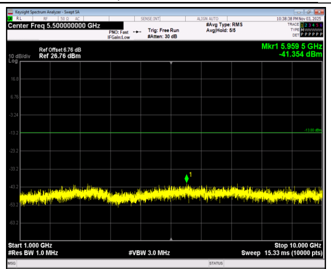
Band5-10MHz-QPSK-20450-1RB#0-Range2:1000~1 0000MHz
