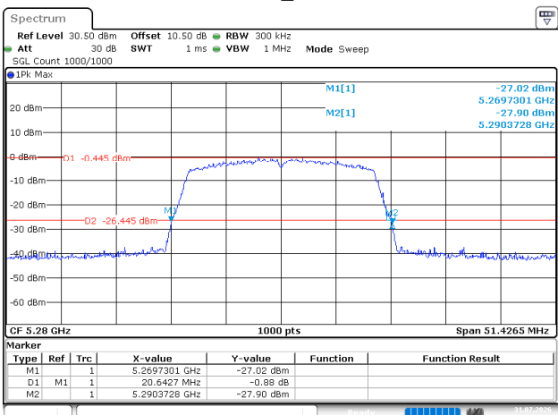
802.11ac20_5280MHz
