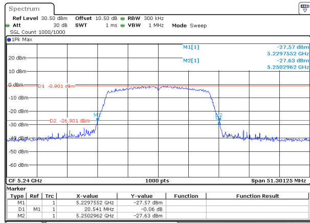
802.11ac20_5240MHz
