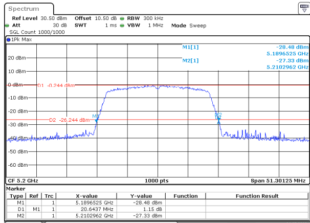
802.11ac20_5200MHz
