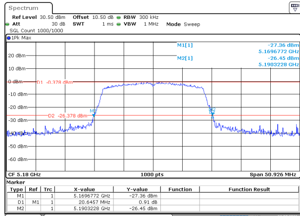
802.11ac20_5180MHz
