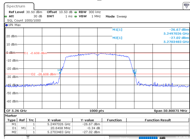
802.11ac20_5260MHz
