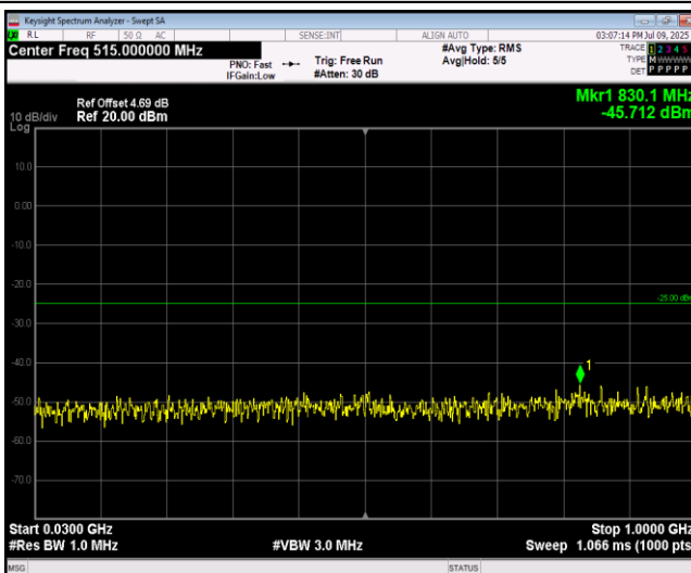
Band12-1.4MHz-QPSK-23017-1RB#0-Range1:30~1000MHz
