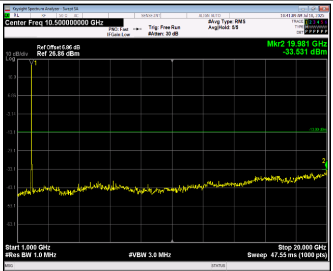
Band25-20MHz-QPSK-26590-1RB#0-Range2:1000~20000MHz
