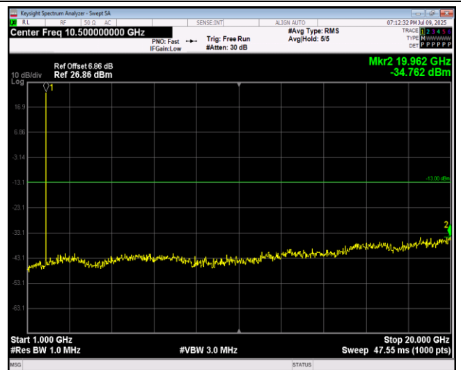
Band25-1.4MHz-64QAM-26365-1RB#0-Range2:1000 ~20000MHz
