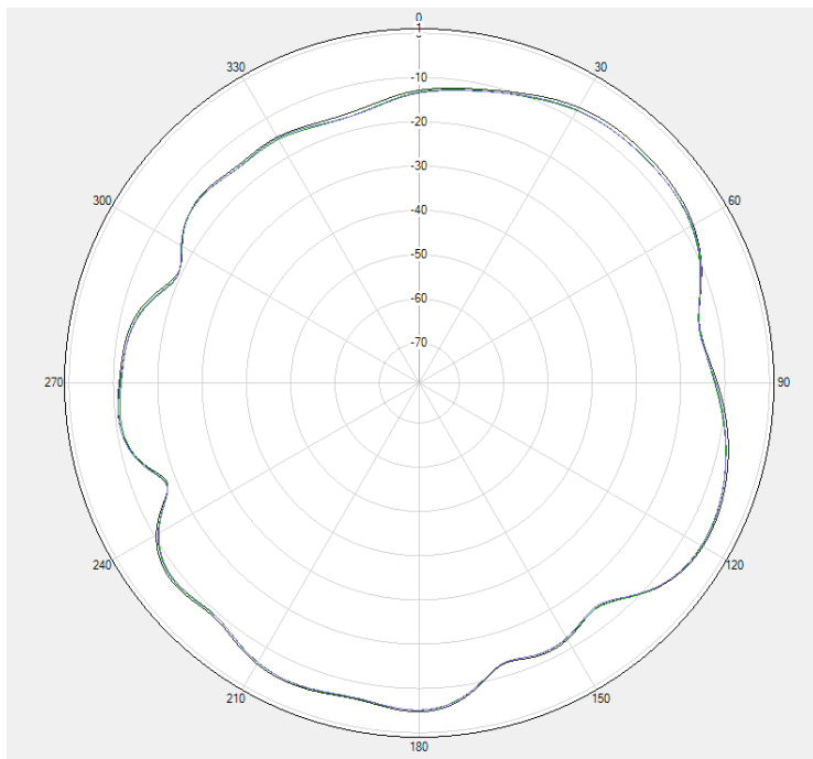
GPS Phi=0deg
