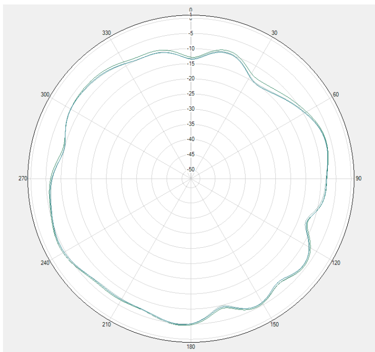
GPS Phi=90deg
