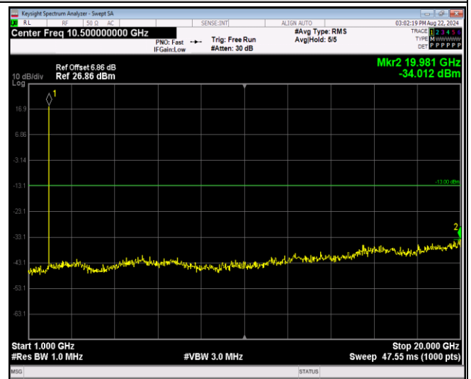
Band2-20MHz-QPSK-18700-1RB#0-Range2:1000~20000MHz
