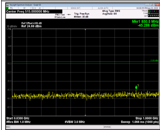
Band2-20MHz-16QAM-19100-1RB#0-Range1:30~100 OMHz
