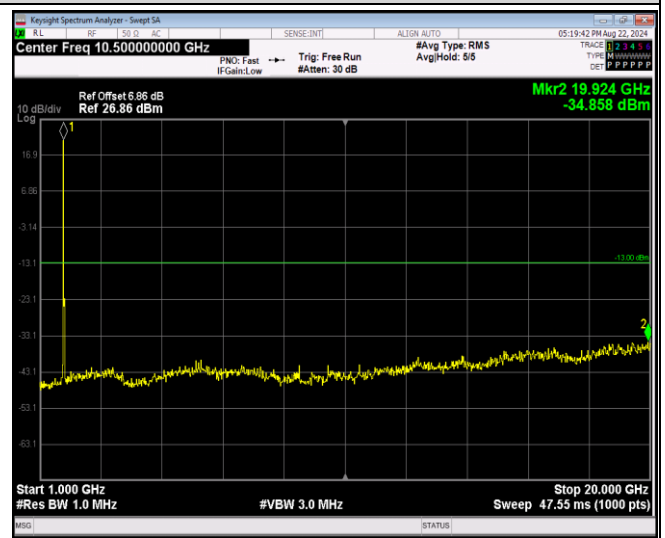
Band4-20MHz-QPSK-20300-1RB#0-Range2:1000~20000MHz
