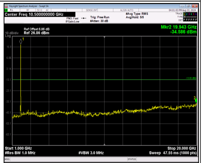
Band2-20MHz-16QAM-19100-1RB#0-Range2:1000~ 20000MHz
