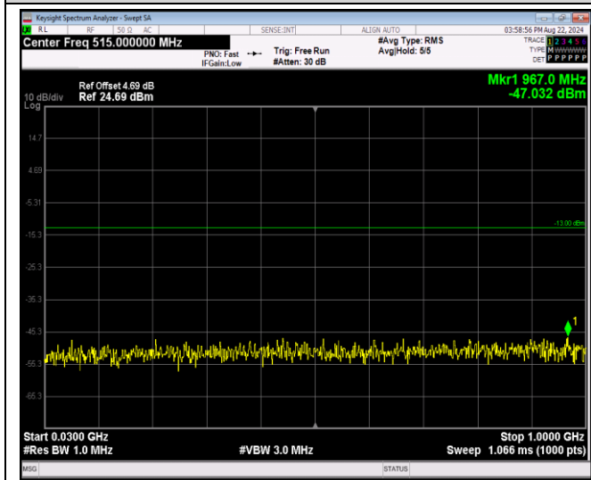
Band2-20MHz-QPSK-18700-1RB#0-Range1:30~1000MHz
