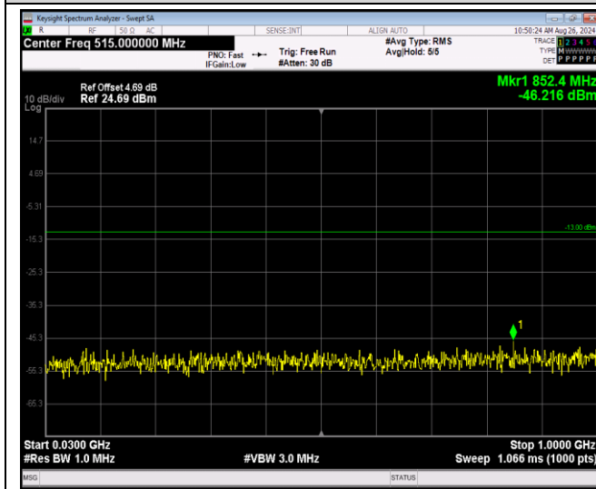
Band4-1.4MHz-QPSK-20175-1RB#0-Range1:30~100 0MHz
