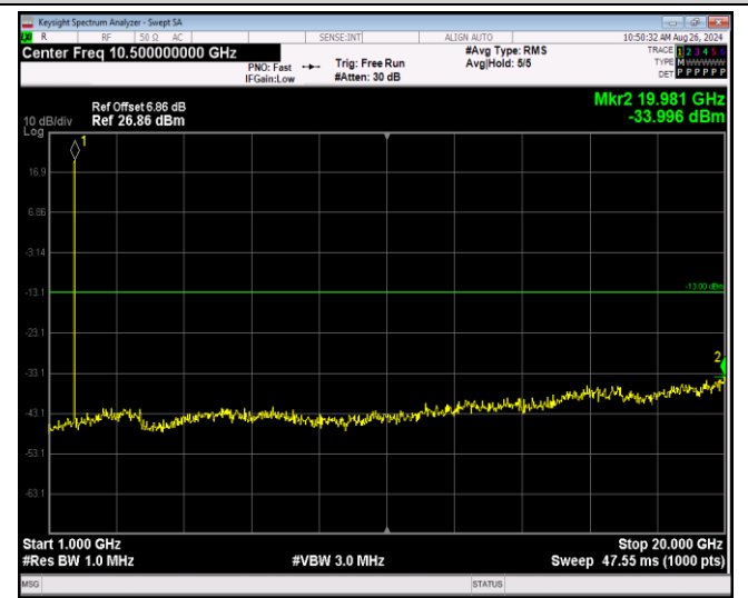
Band4-1.4MHz-QPSK-20175-1RB#0-Range2:1000~20 000MHz
