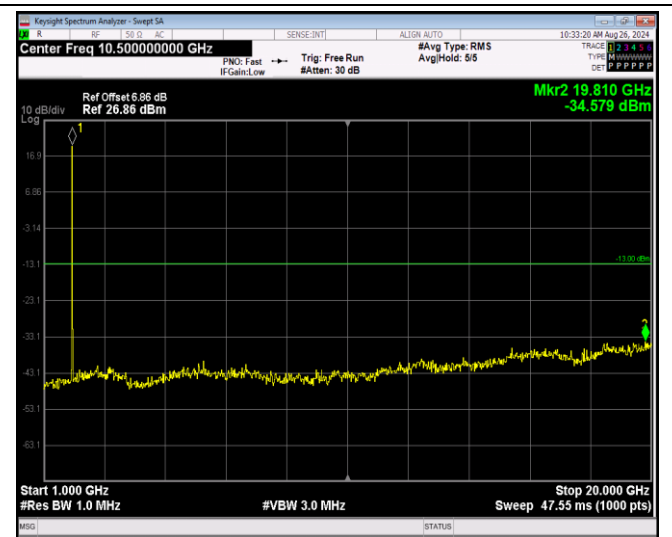
Band4-1.4MHz-QPSK-19957-1RB#0-Range2:1000~20 000MHz
