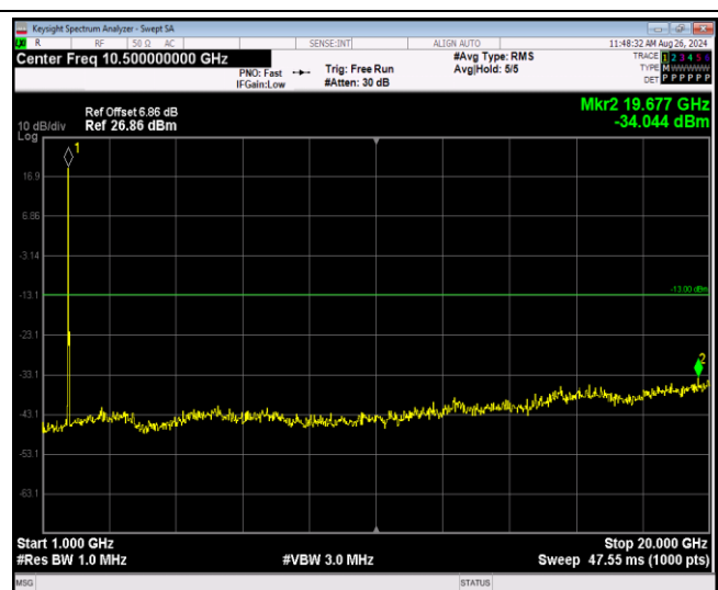
Band4-20MHz-64QAM-20050-1RB#0-Range2:1000~2 0000MHz
