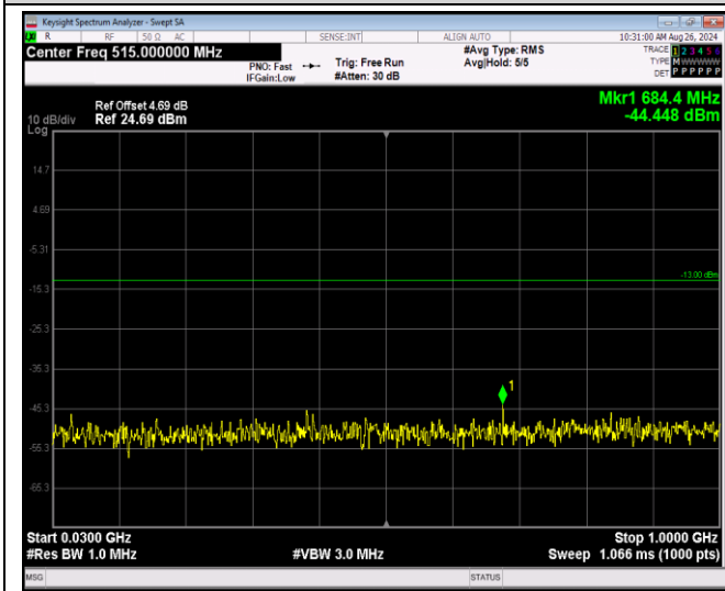
Band2-20MHz-QPSK-18700-1RB#0-Range1:30~1000MHz
