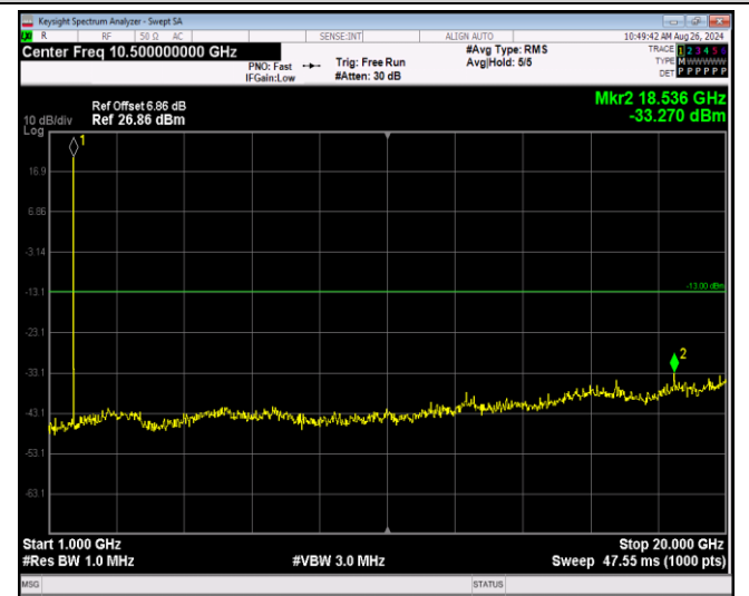
Band4-1.4MHz-QPSK-20175-1RB#0-Range2:1000~20 000MHz
