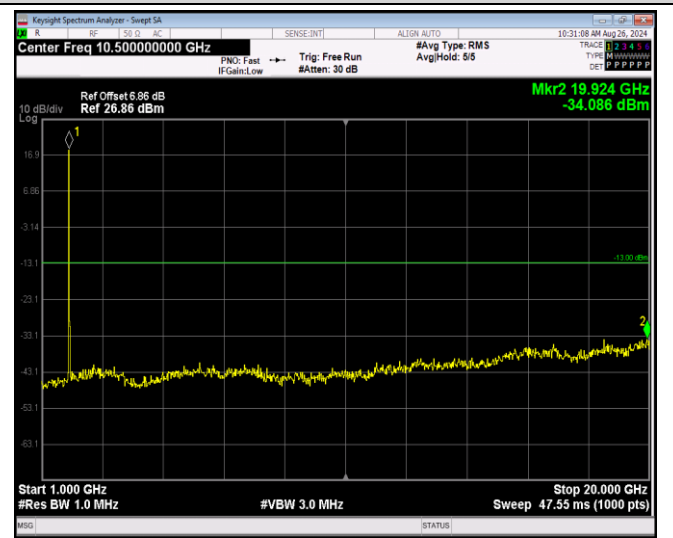
Band2-20MHz-QPSK-18700-1RB#0-Range2:1000~20000MHz
