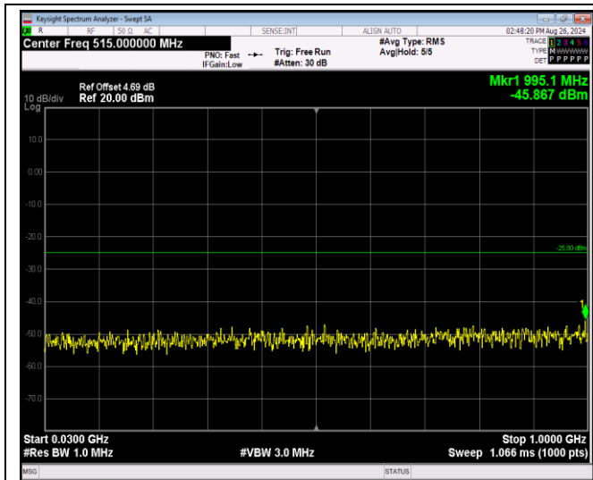
Band41-20MHz-QPSK-41140-1RB#0-Range1:30~100 OMHz
