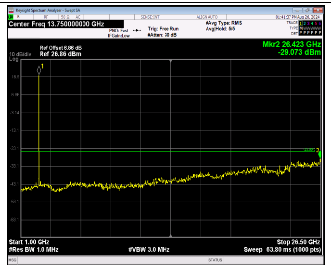
Band7-20MHz-16QAM-21350-1RB#0-Range2:1000~2 6500MHz
