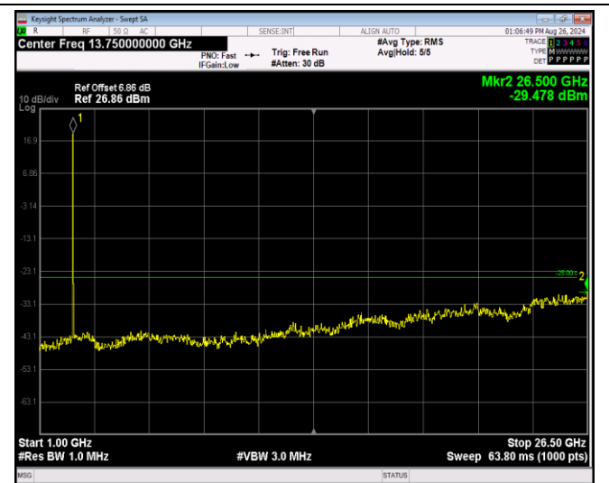
Band7-20MHz-QPSK-20850-1RB#0-Range2:1000~26 500MHz
