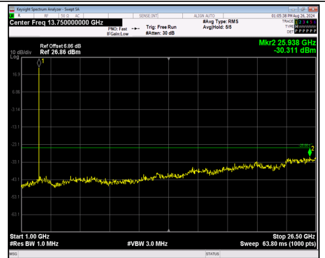
Band7-5MHz-16QAM-21425-1RB#0-Range2:1000~26 500MHz
