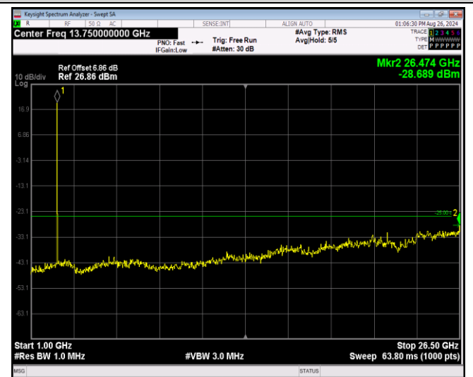
Band7-5MHz-16QAM-21425-1RB#0-Range2:1000~26 500MHz
