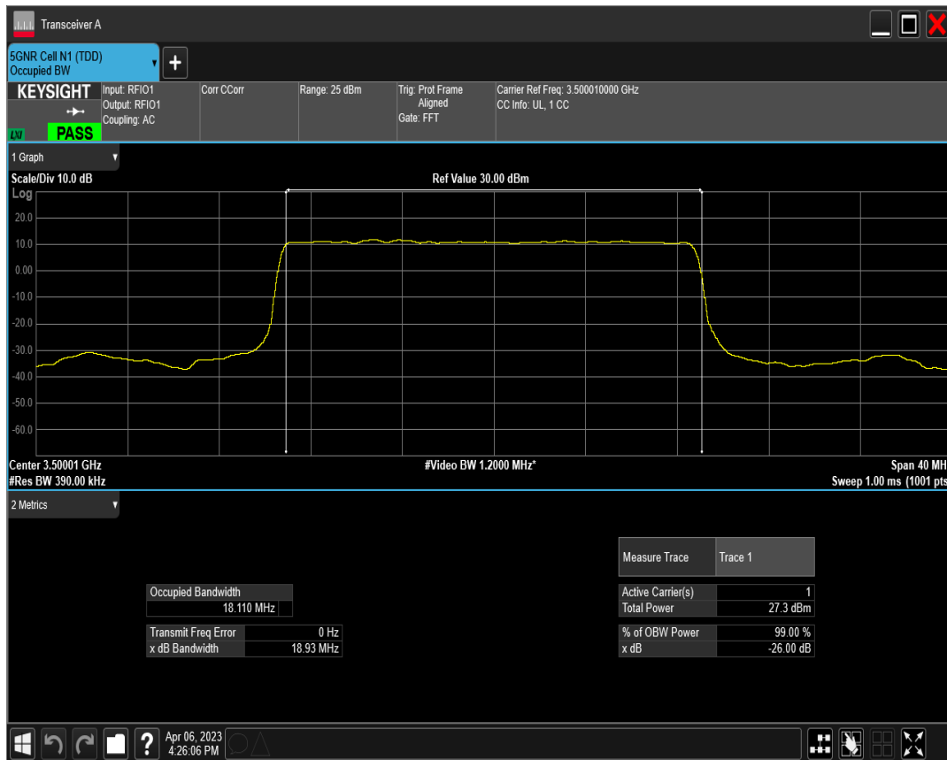
n77(3450-3550) SCS=30kHz DFT_QPSK BW=20MHz Channel=633334 RB=50@0
