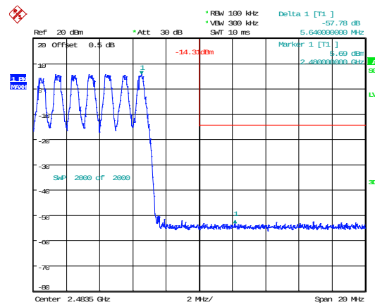
DH1_Hopping_Upper
