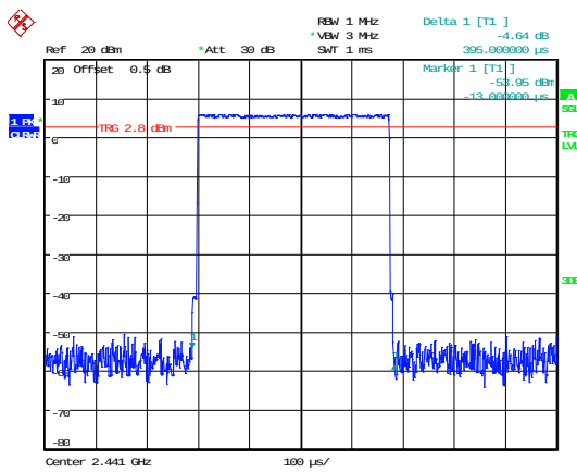
DH1_Hopping
