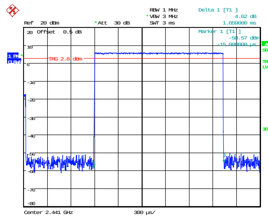
DH3_Hopping
