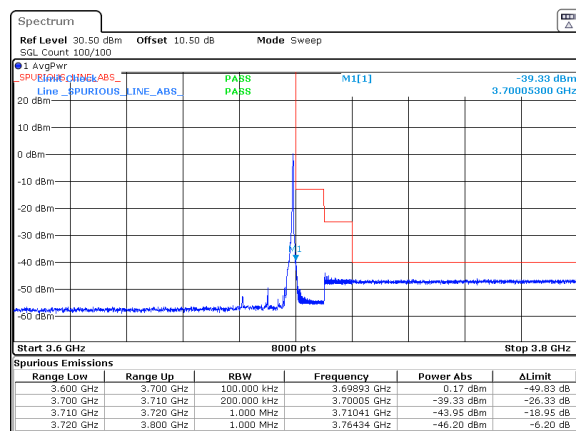
n77_2_20MHz_30kHz_3690MHz_DFT-s-OFDM QPSK_RB1@50
