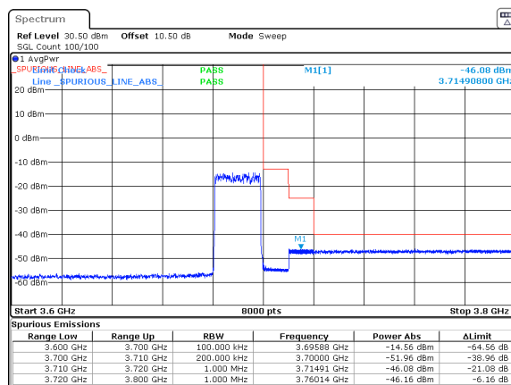
n77_2_20MHz_30kHz_3690MHz_DFT-s-OFDM QPSK_RB50@0
