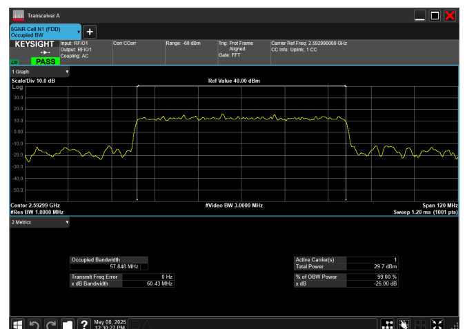
n41_60MHz_30kHz_2592.99MHz_CP-OFDM QPSK_RB162@0
