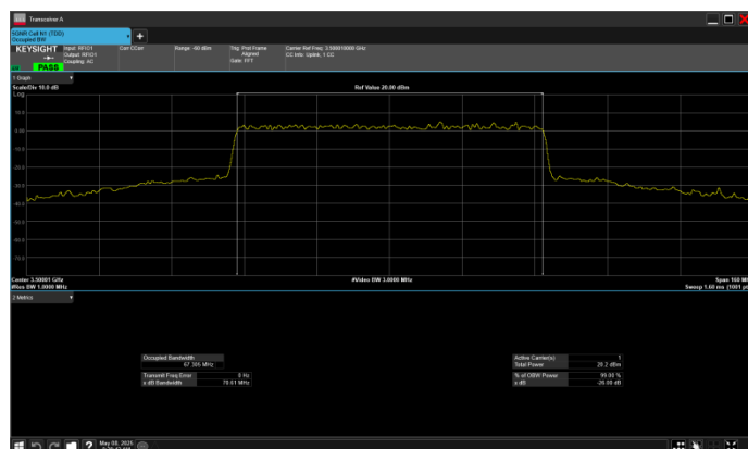
n77_1_70MHz_30kHz_3500MHz_CP-OFDM QPSK_RB189@0
